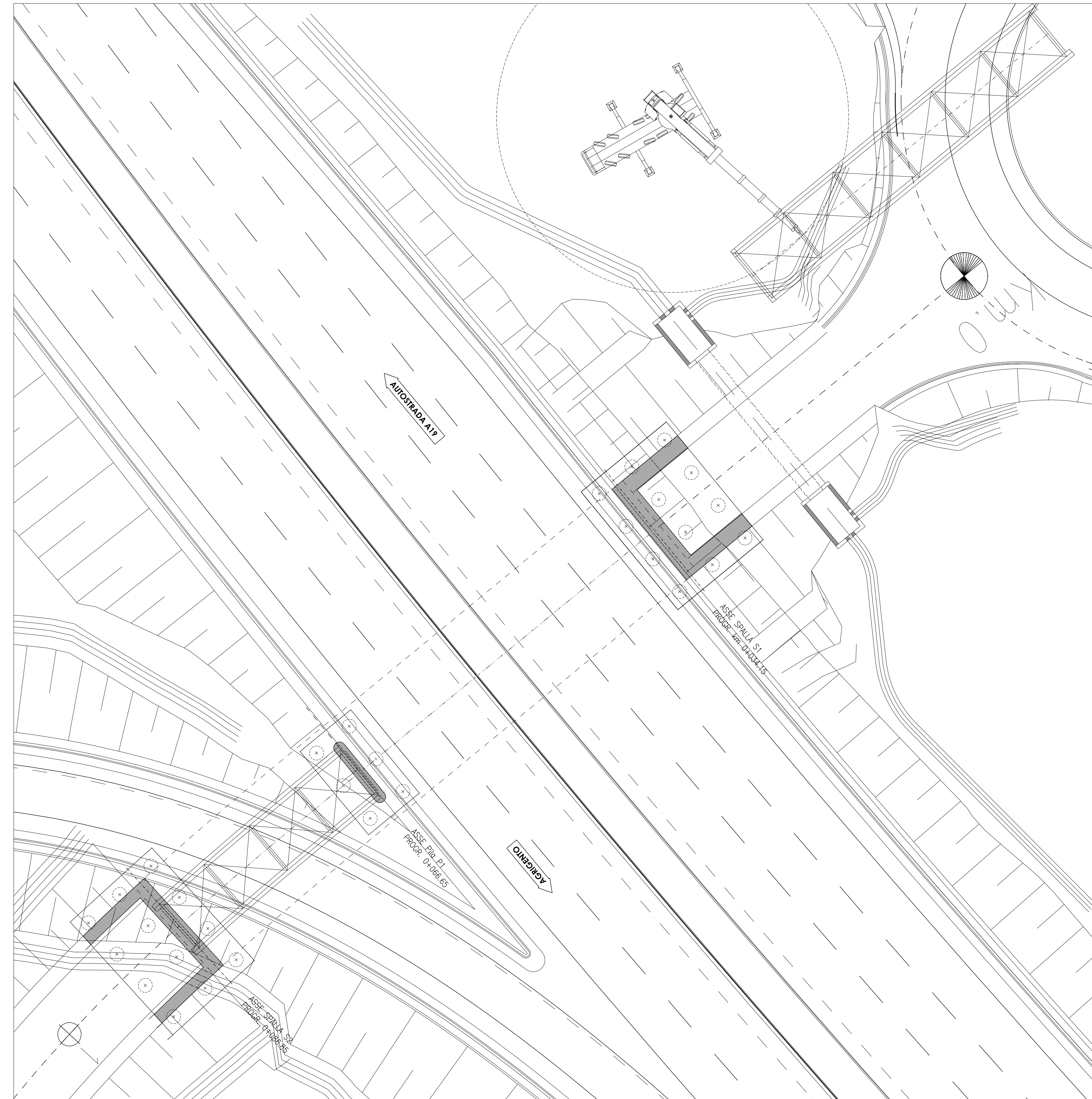
FASE COSTRUTTIVA 02
