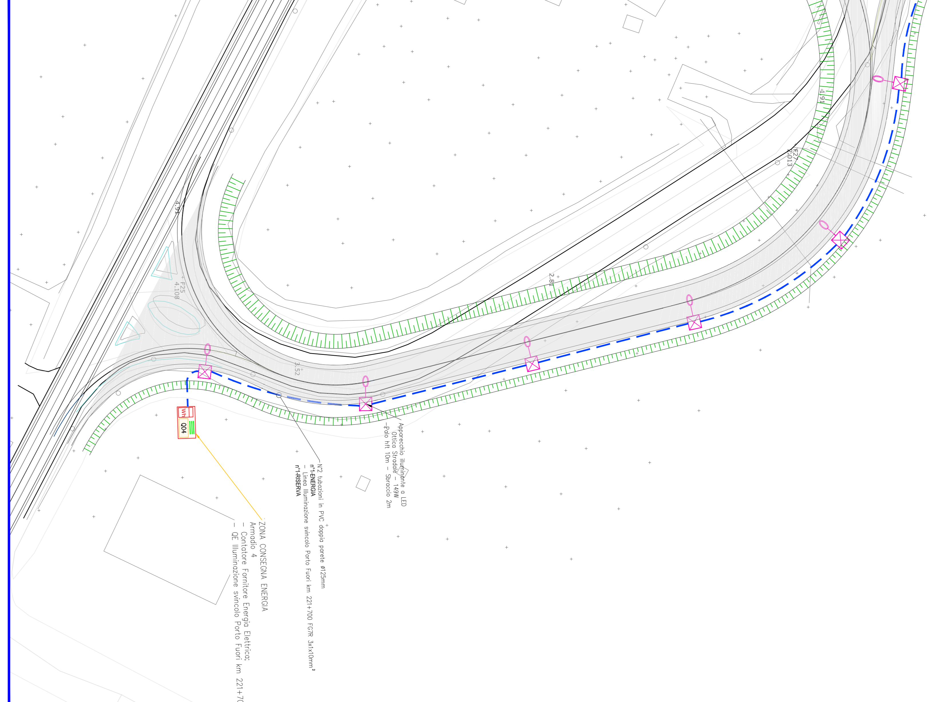
DETTAGLIO 2 (scala 1:500)
