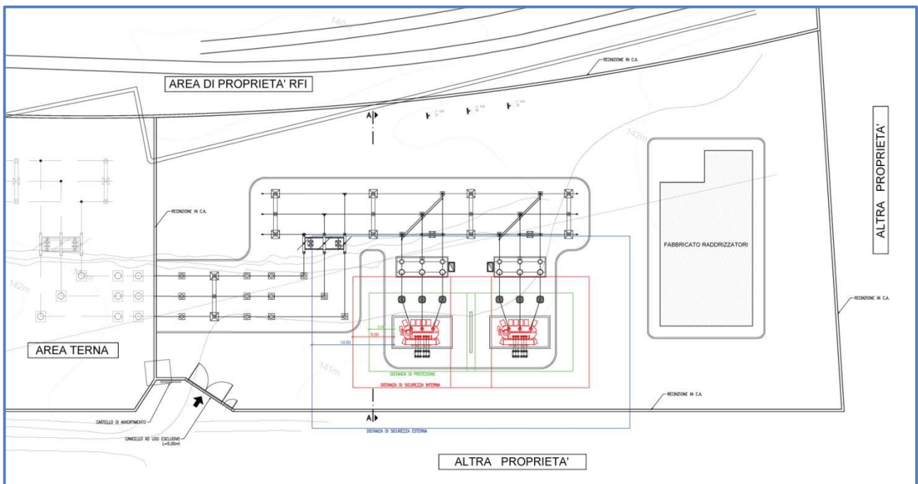
Planimetria del piazzale della nuova SSE di PARTINICO
