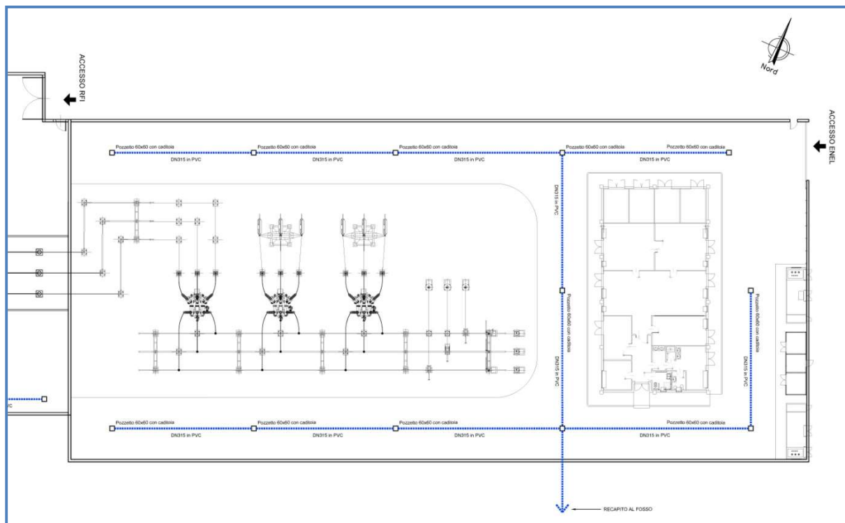
Planimetria futuro piazzale ENEL
