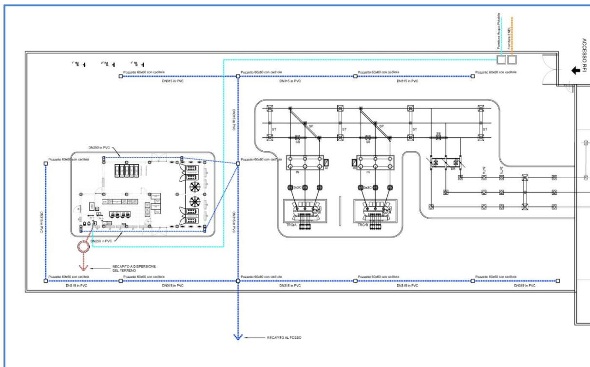
Planimetria piazzale RFI
