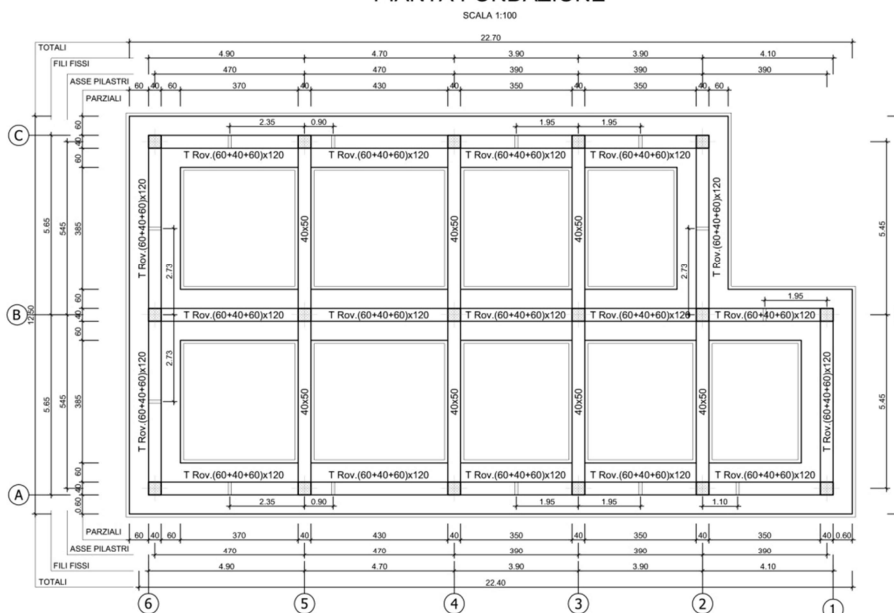
PIANTA FONDAZIONE
