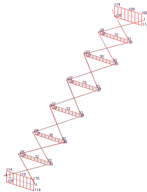
Inviluppo Taglio
