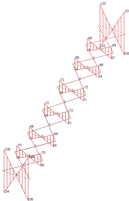
Inviluppo Momento
