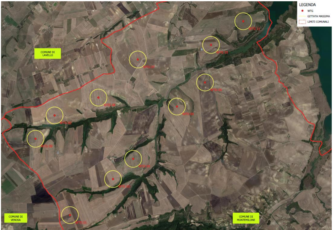
Figura 1 - Gittata massima della pala in caso di distacco - planimetria
