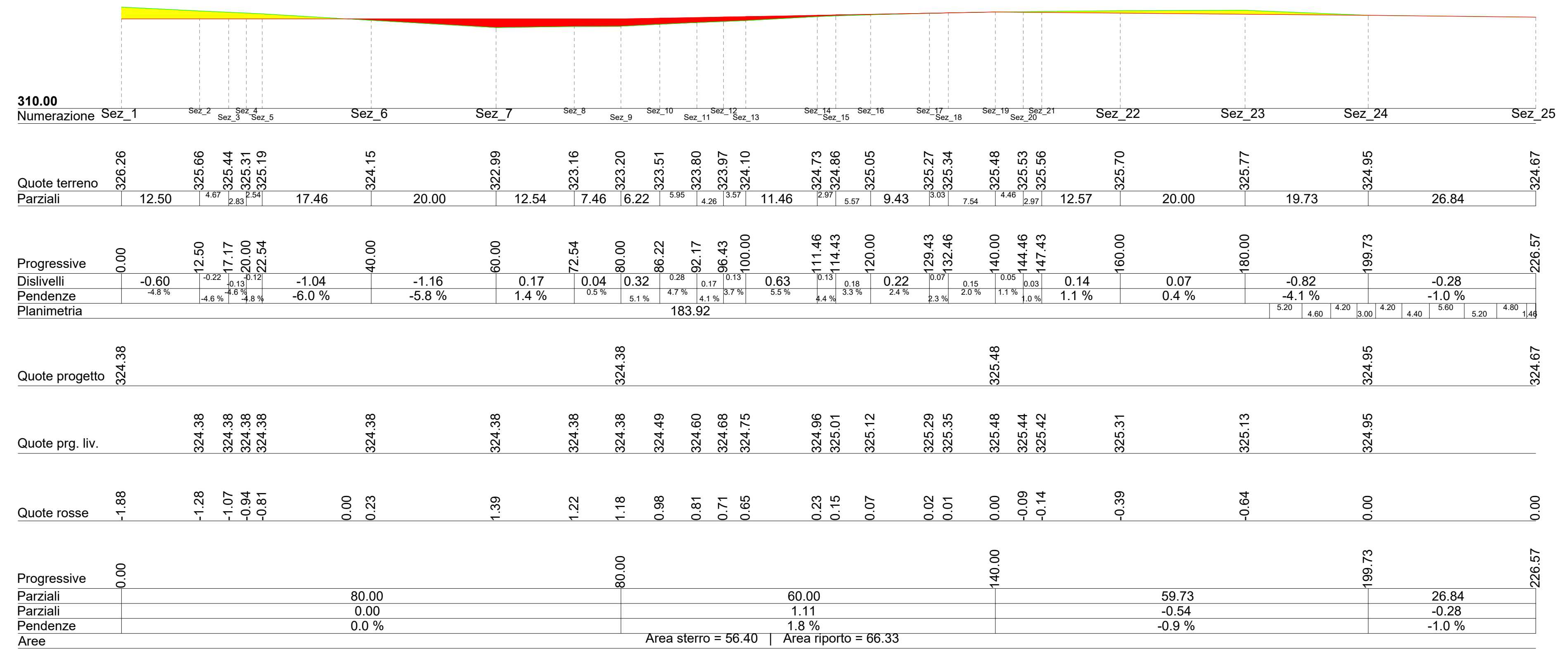
PROFILO LONGITUDINALE WTG 03 scala 1:500
