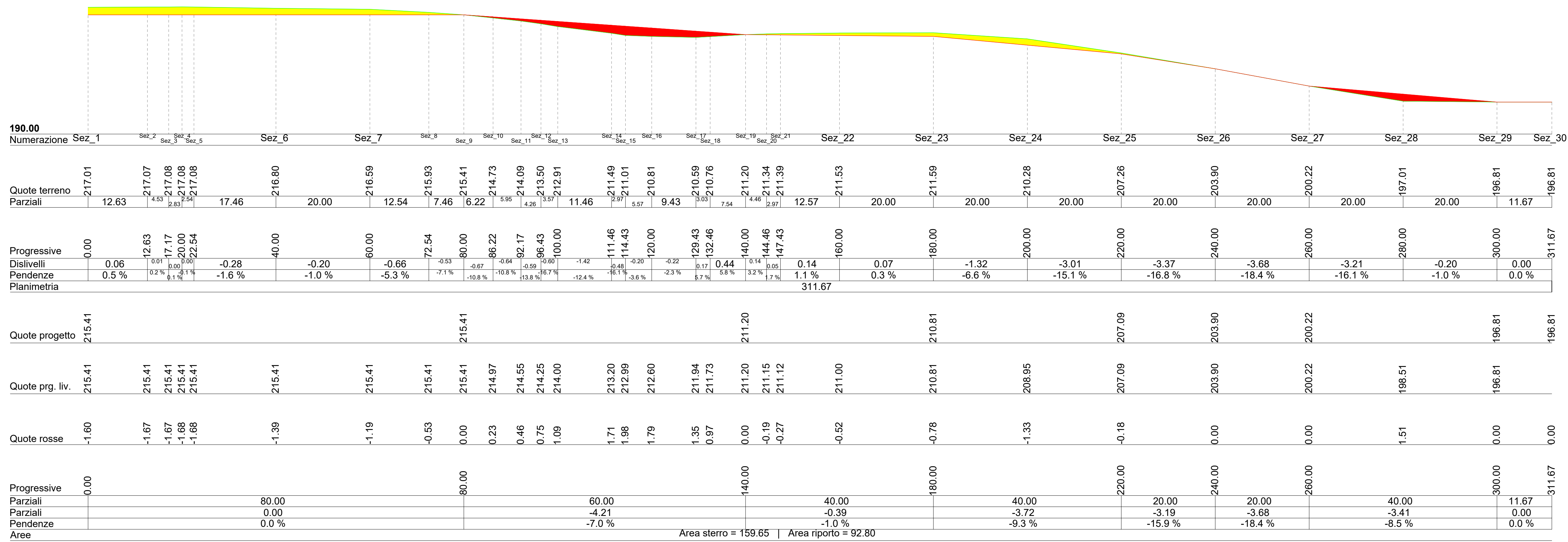
PROFILO LONGITUDINALE WTG 06 scala 1:500
