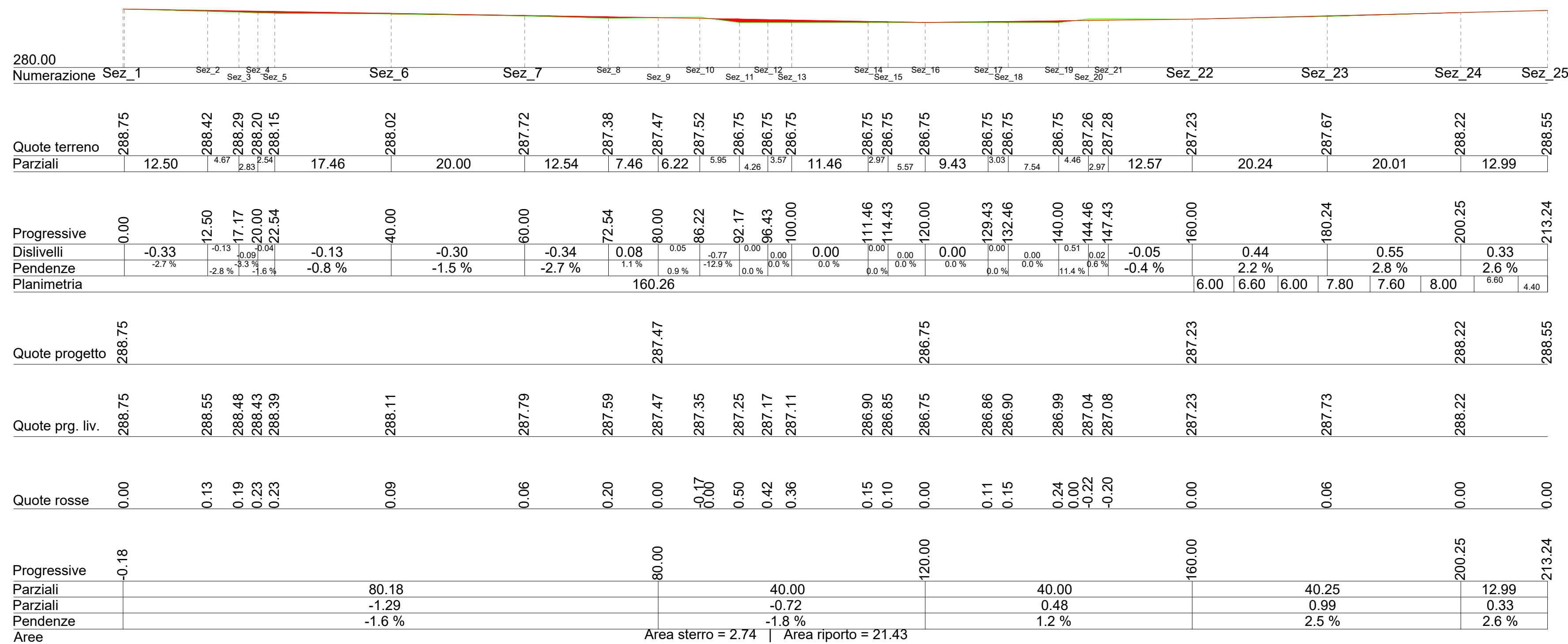
PROFILO LONGITUDINALE WTG 07 scala 1:500
