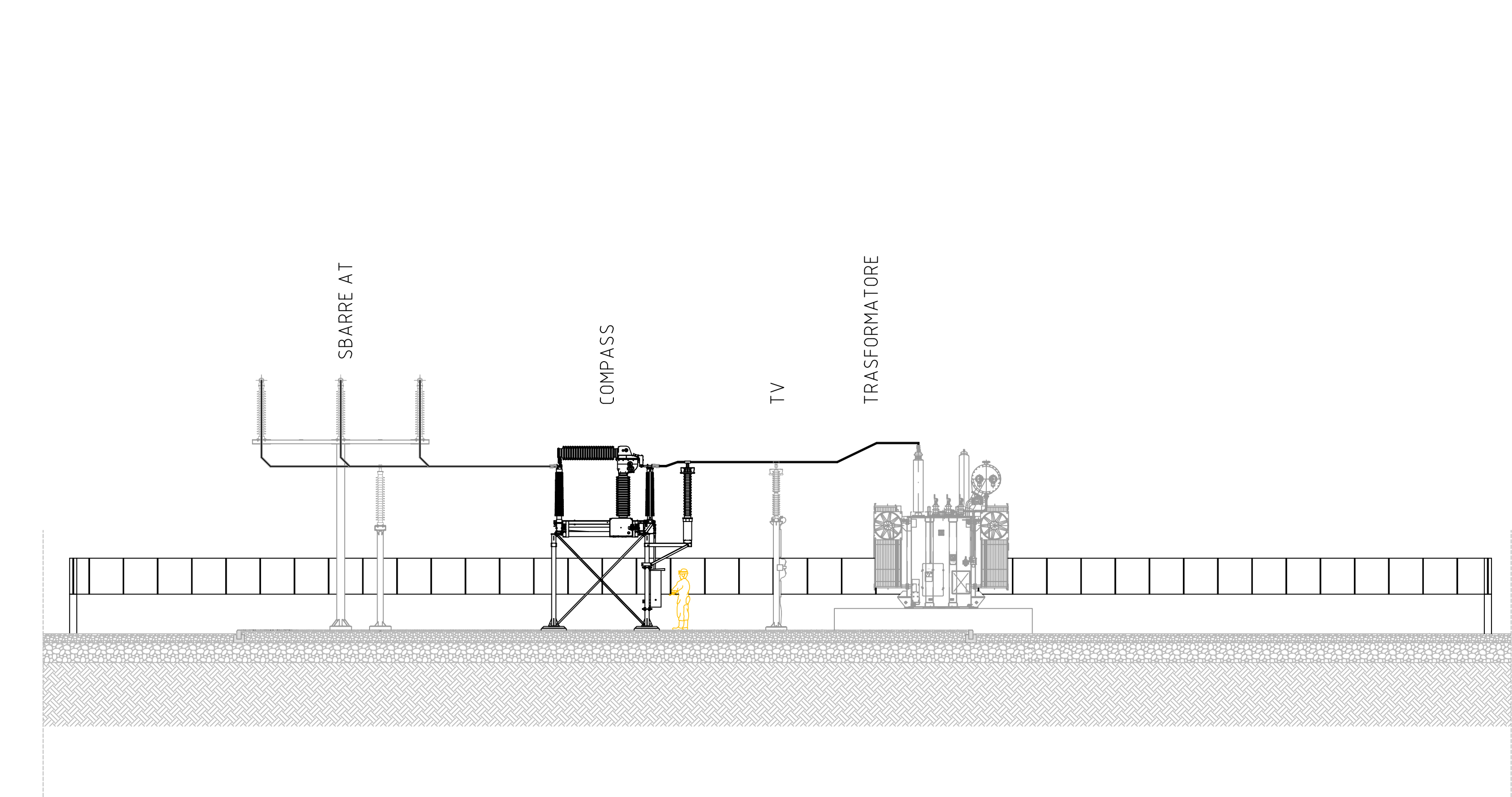
Stazione di Utanza - Sezioni longitudinali Scala 1:100
