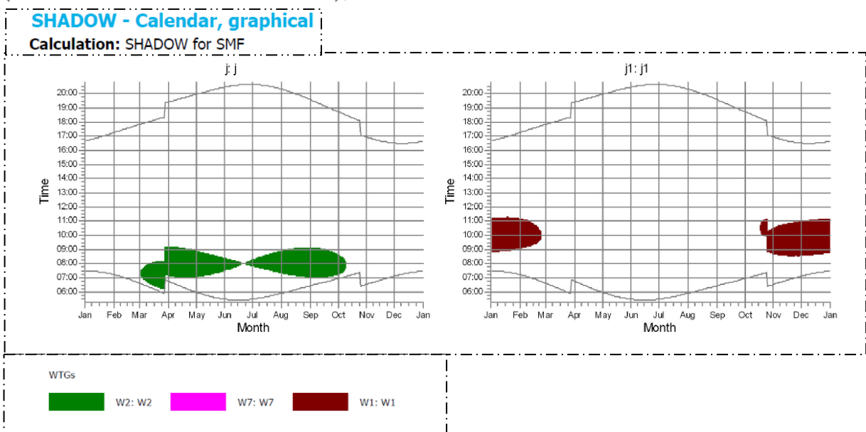
Figura 13: riquadro preso dal CALENDAR grafico e relativo ai ricettori R1 ed R2
