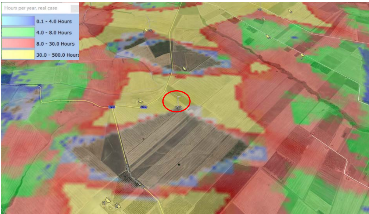
Figura 11: inquadramento sul ricettore R-J soggetto al fenomeno di ombreggiamento da parte della WTG02
