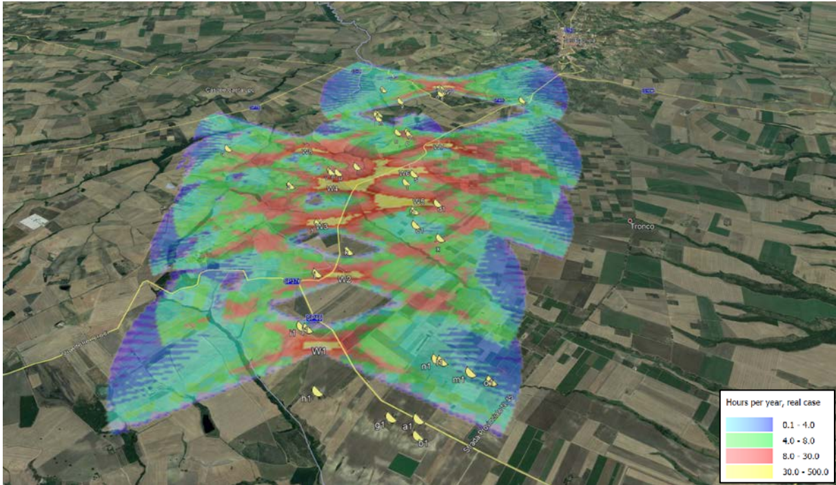
Figura 15: mappa del real case
