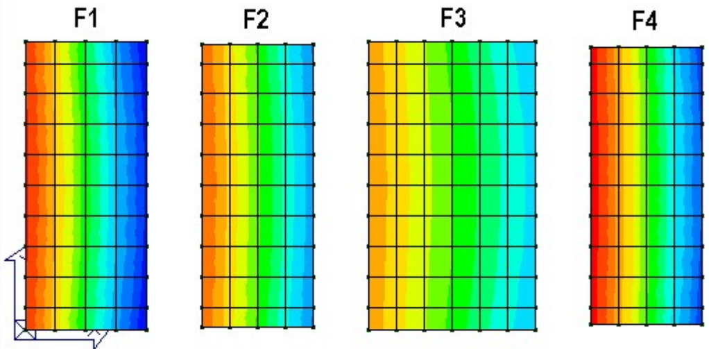
Mapa cromatica delle pressioni sul terreno - Comb. SLE rara
