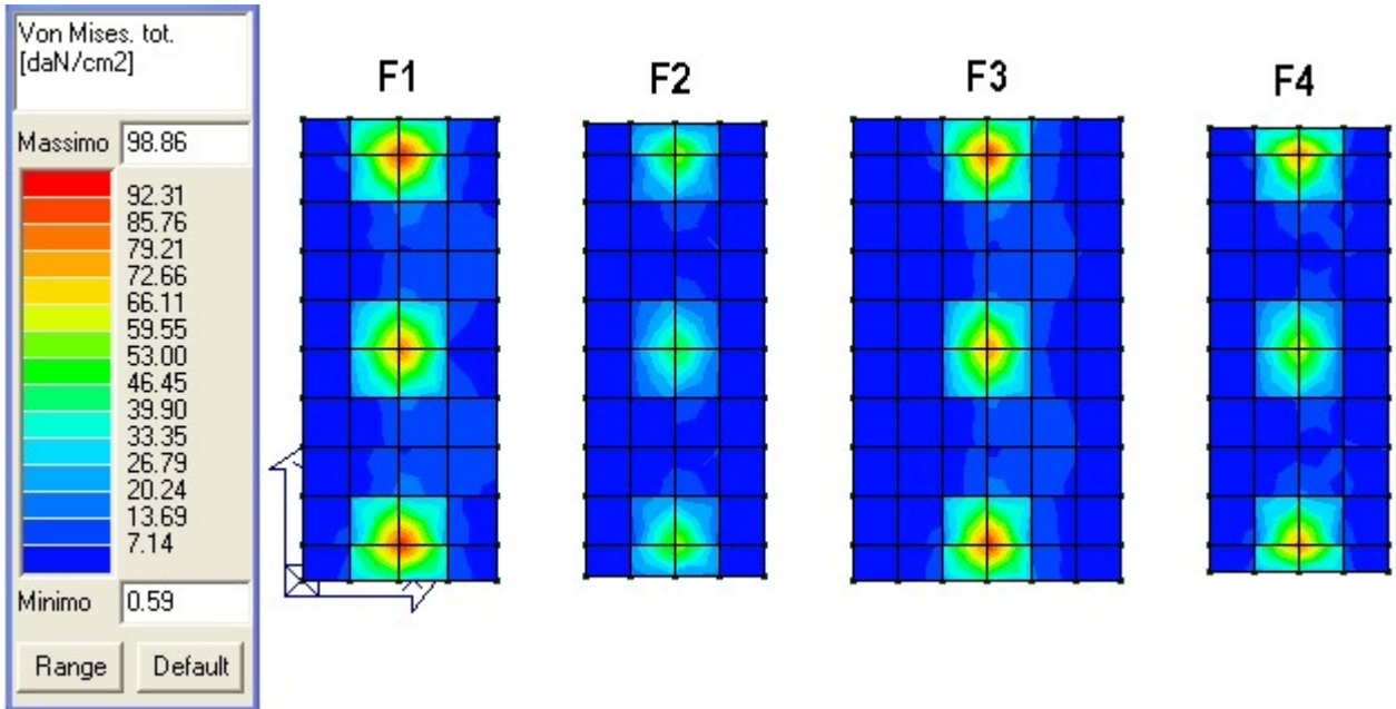
Mapa cromatica delle tensioni totali (membrana + flessione) ottenute mediante la formulazione di Von Mises - Comb. SLU
