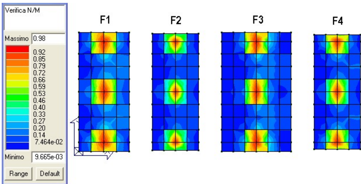
Rapporto S_d/S_u
