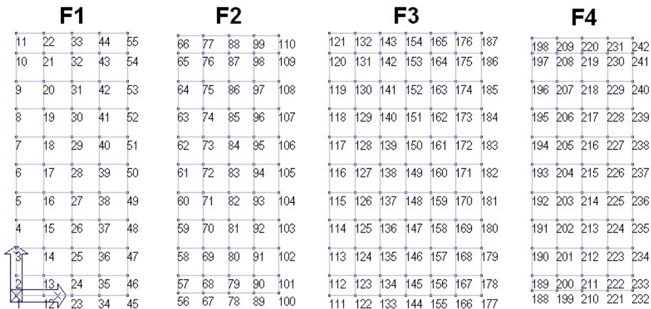
Modello F.E.M. – Numerazione nodi
