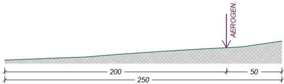
SEZIONE DI VERIFICA WTG1 - POST OPERA
