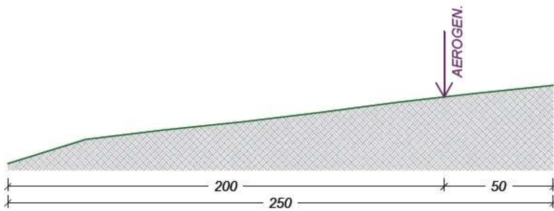
SEZIONE DI VERIFICA WTG3 - POST OPERA
