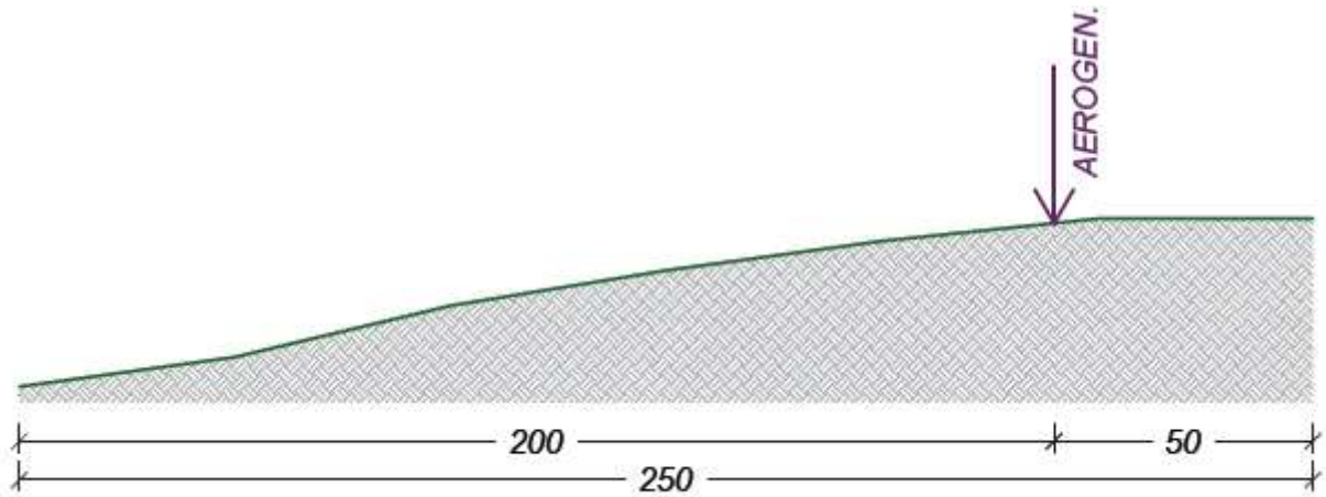
SEZIONE DI VERIFICA WTG6 - POST OPERA
