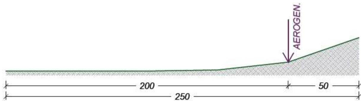
SEZIONE DI VERIFICA WTG4 - POST OPERA
