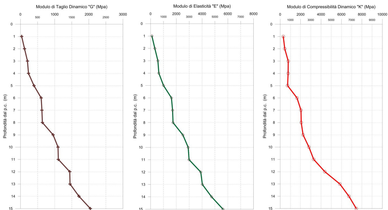
Fig. 2.4.16 - A sinistra, diagramma relativo all'andamento del modulo elastico "G" in funzione della profondità dal p.c. Al centro, diagramma relativo all'andamento del modulo elastico "E" in funzione della profondità dal p.c. A destra, diagramma relativo all'andamento del modulo elastico "K" in funzione della profondità dal p.c.
