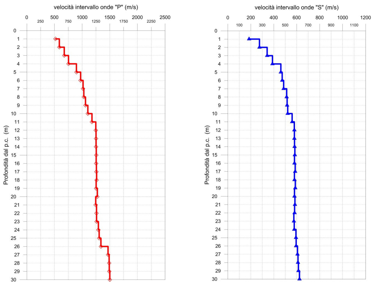
Fig. 2.4.2 - A sinistra, diagramma relativo all'andamento delle velocità intervallo delle onde "P", in funzione della profondità dal p.c.
