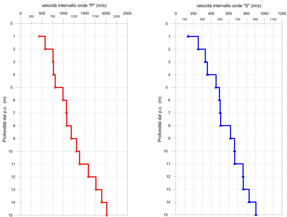
Fig. 2.4.14 - A sinistra, diagramma relativo all'andamento delle velocità intervallo delle onde "P", in funzione della profondità dal p.c.
