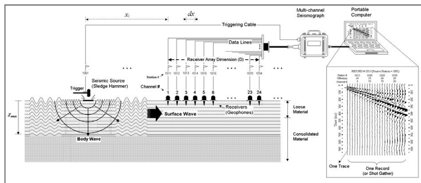
Fig. 3.1.1 – Esempio configurazione sorgente-ricevitori per l'esecuzione di un rilievo MASW.
