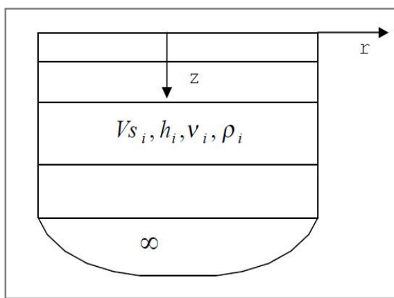
Fig. 3.1.2 - Modello di semispazio semplificato.
