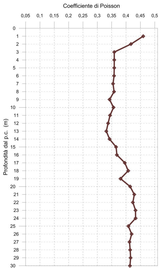
Fig. 2.4.11 - Diagramma relativo all'andamento del coefficiente di Poisson in funzione della profondità dal p.c.
