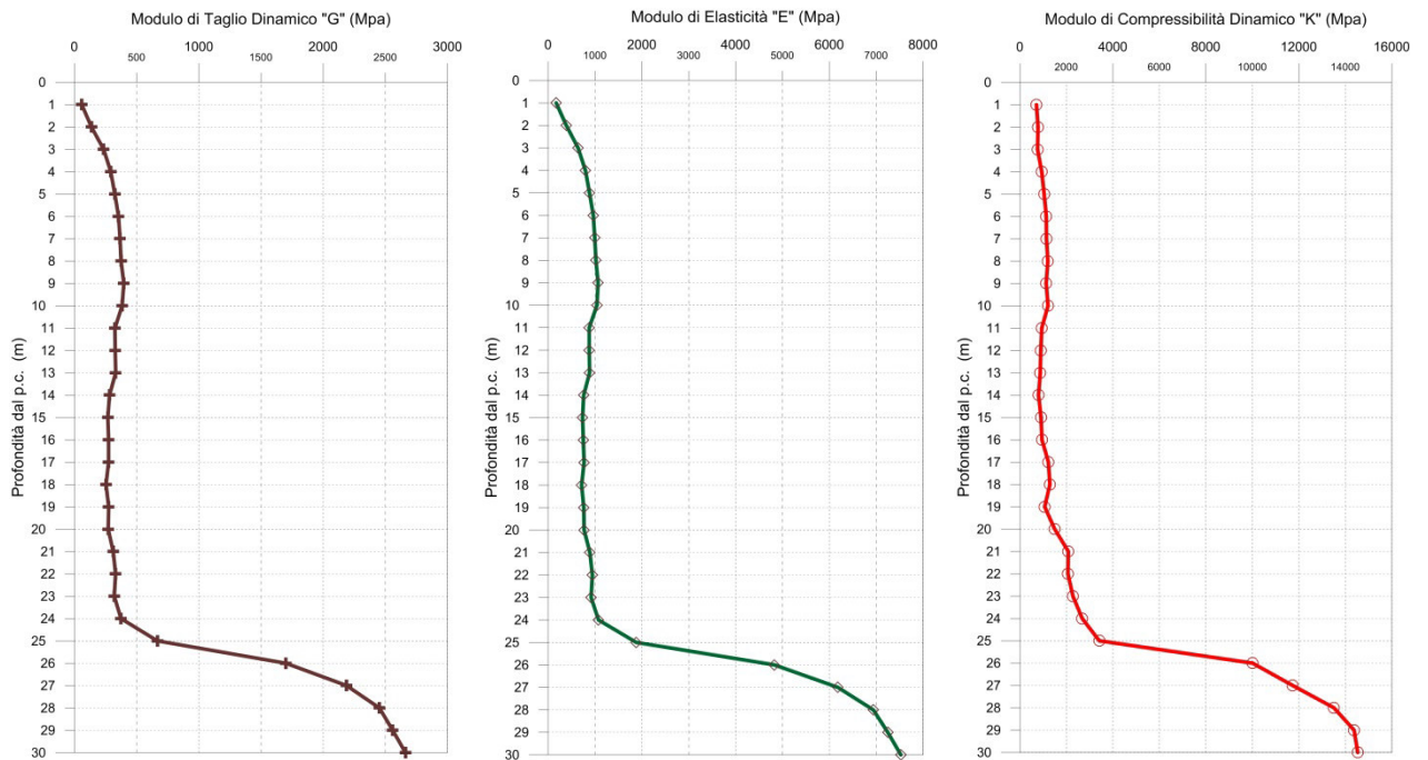
Fig. 2.4.12 - A sinistra, diagramma relativo all'andamento del modulo elastico "G" in funzione della profondità dal p.c. Al centro, diagramma relativo all'andamento del modulo elastico "E" in funzione della profondità dal p.c. A destra, diagramma relativo all'andamento del modulo elastico "K" in funzione della profondità dal p.c.
