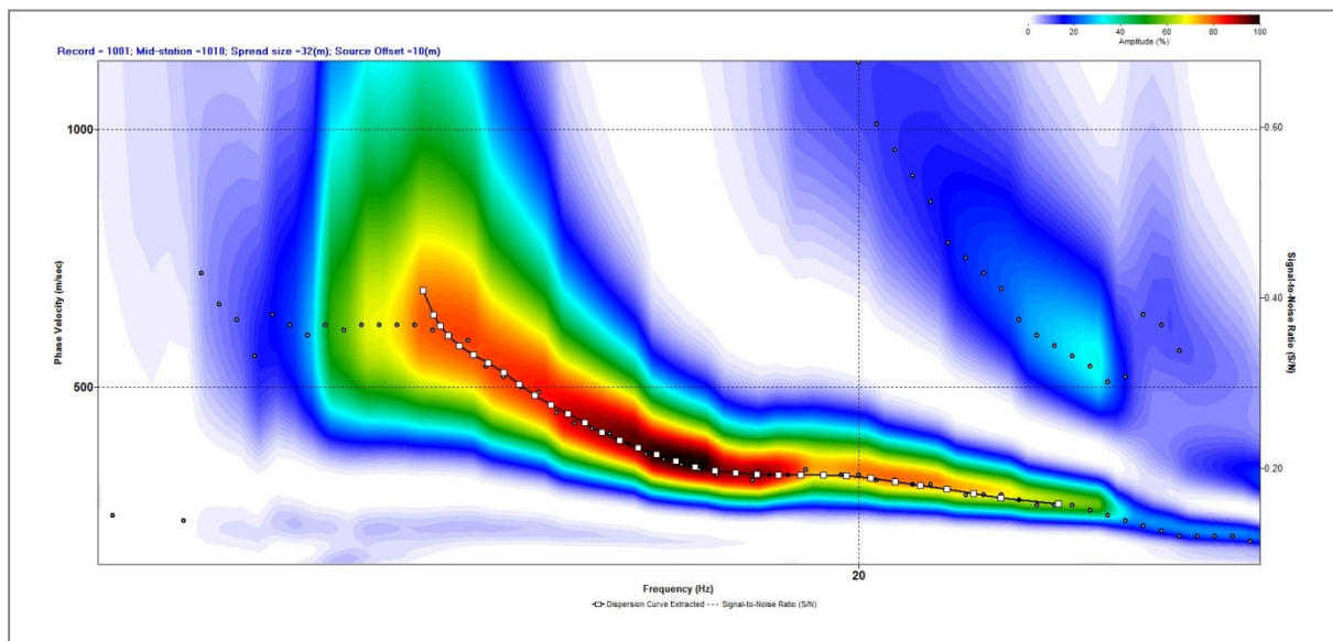
Fig. 3.4.2 - Curva F-K con evidenza del picking dei massimi spettrali.
