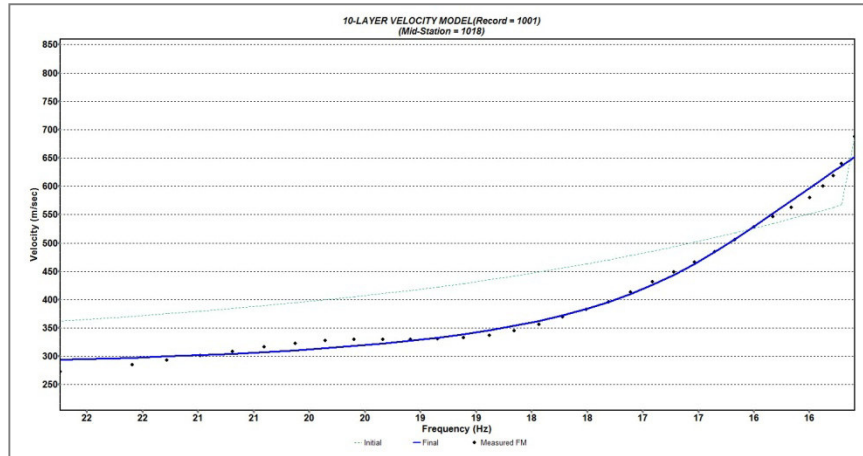
Fig. 3.4.3 - Confronto tra la curva di dispersione stimata e quella sintetica generata dal modello finale di V_S .
