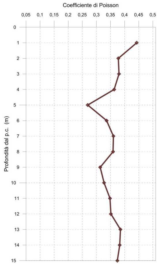
Fig. 2.4.15 - Diagramma relativo all'andamento del coefficiente di Poisson in funzione della profondità dal p.c.
