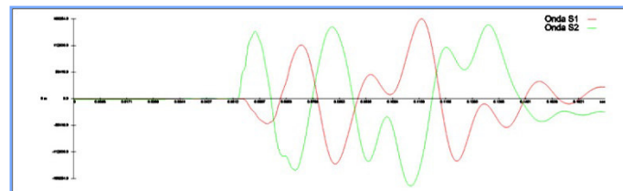
Fig. 2.1.3 - Esempio di onda S e di inversione di fase necessaria per l'individuazione del tempo di arrivo dell'onda di taglio (onda S).
