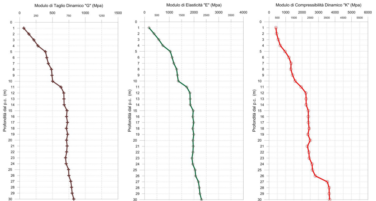
Fig. 2.4.4 - A sinistra, diagramma relativo all'andamento del modulo elastico "G" in funzione della profondità dal p.c. Al centro, diagramma relativo all'andamento del modulo elastico "E" in funzione della profondità dal p.c. A destra, diagramma relativo all'andamento del modulo elastico "K" in funzione della profondità dal p.c.
