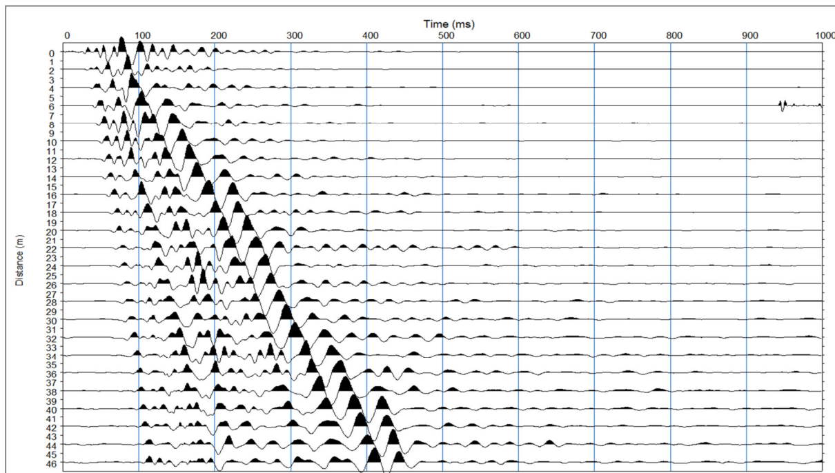
Fig. 3.4.1 - Sismogrammi.
