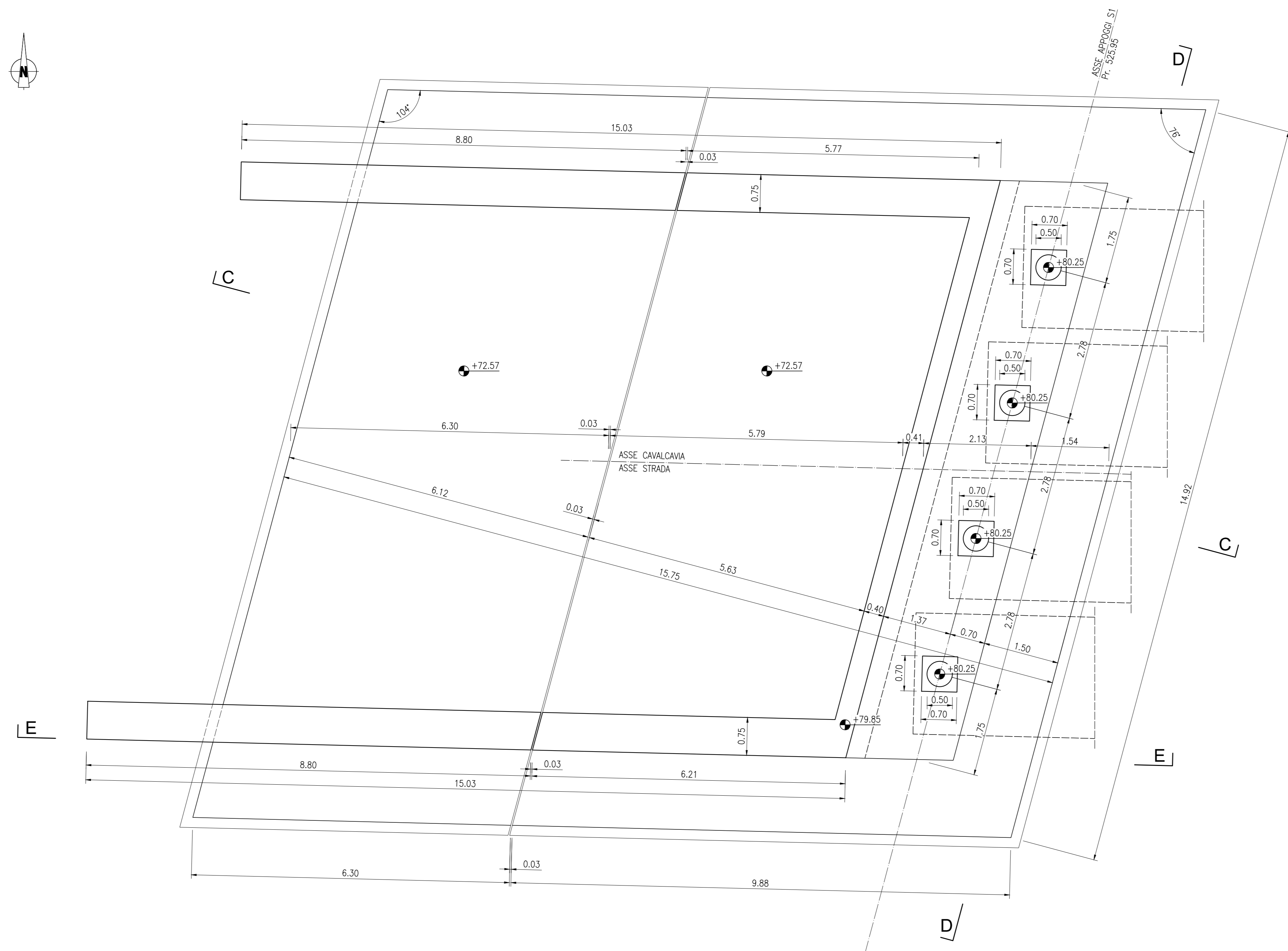
VISTA DALL'ALTO (1:50)
