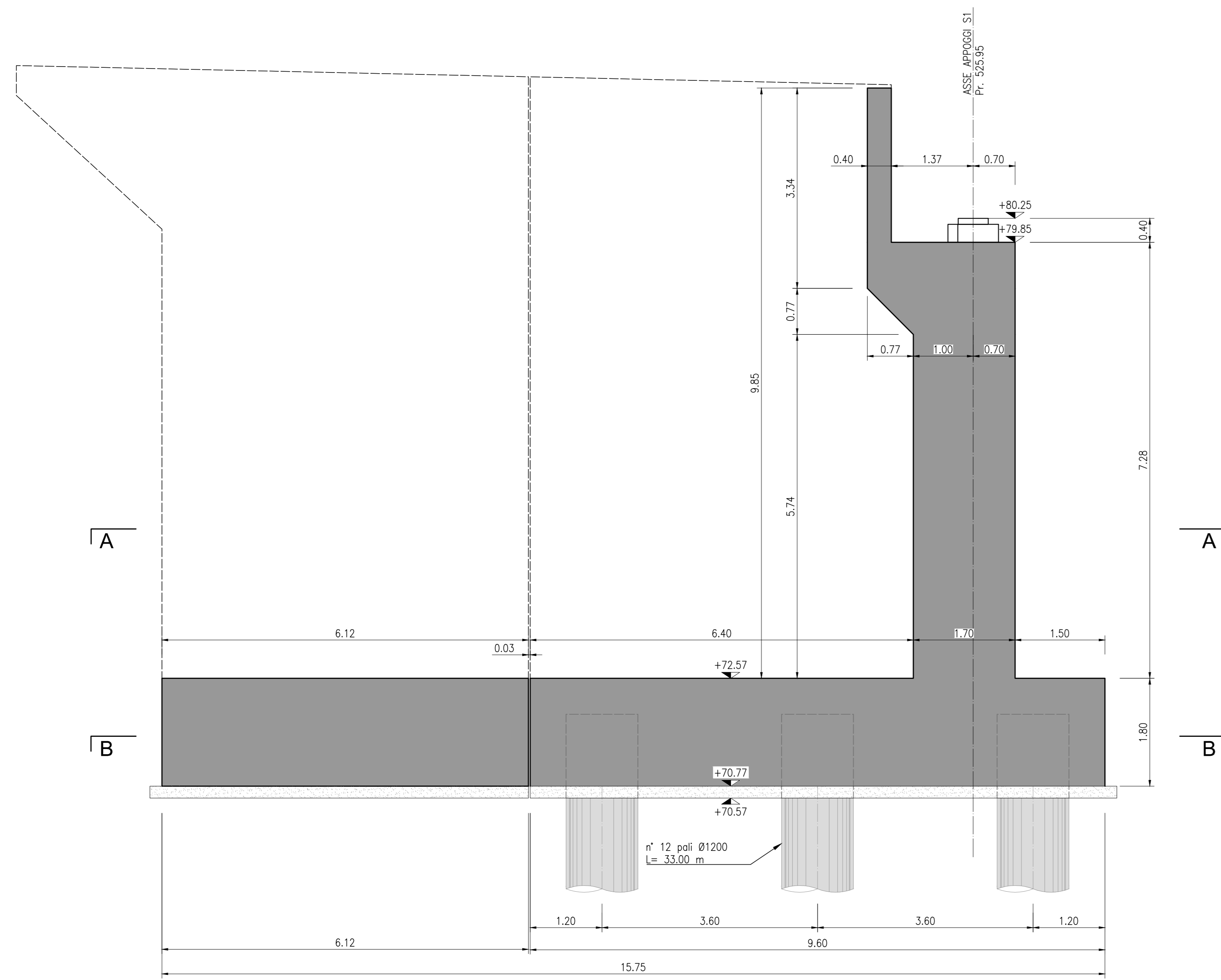
SEZIONE C-C (1:50)
