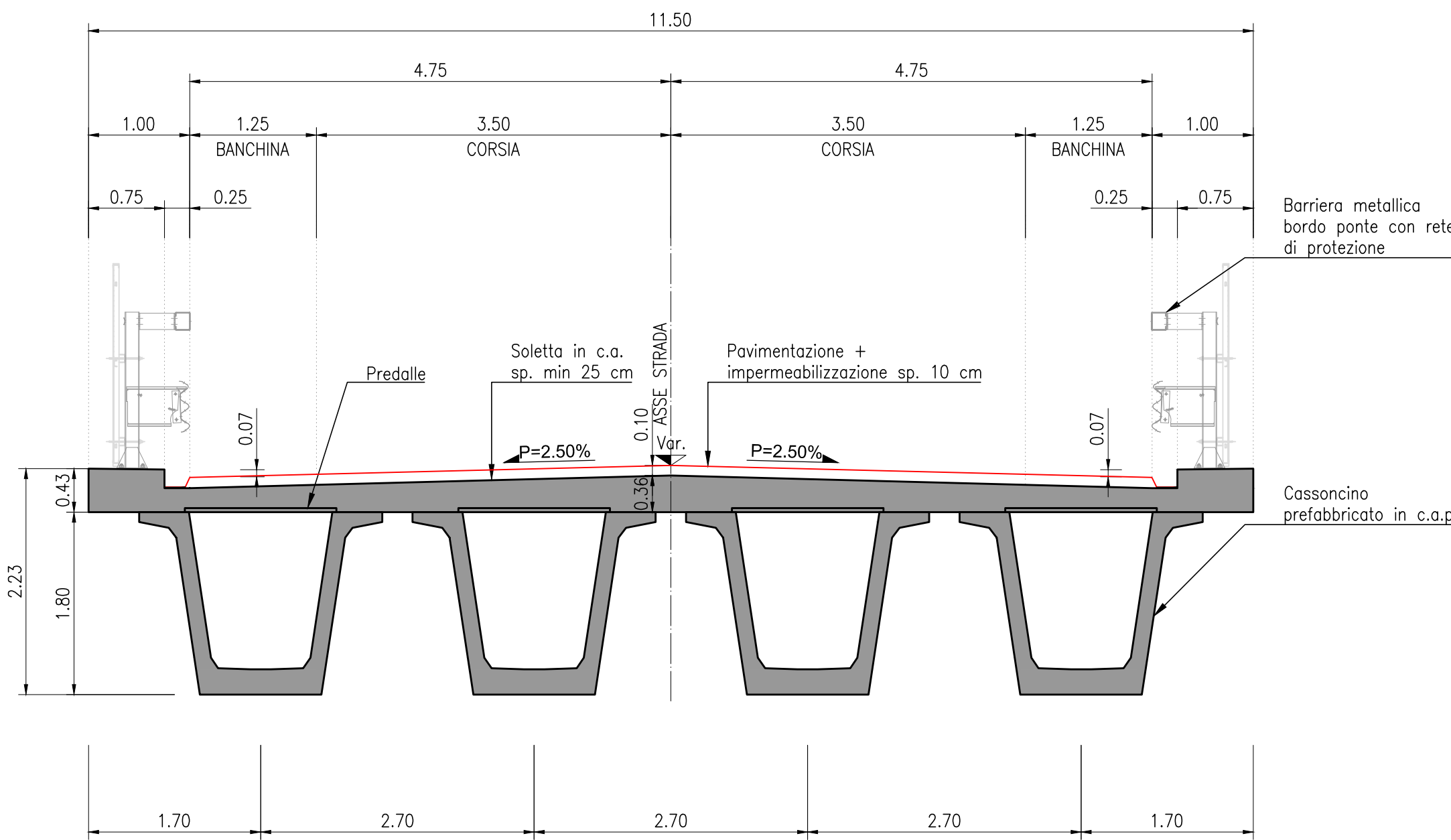
SEZIONE TRASVERSALE TIPO (1:50)
