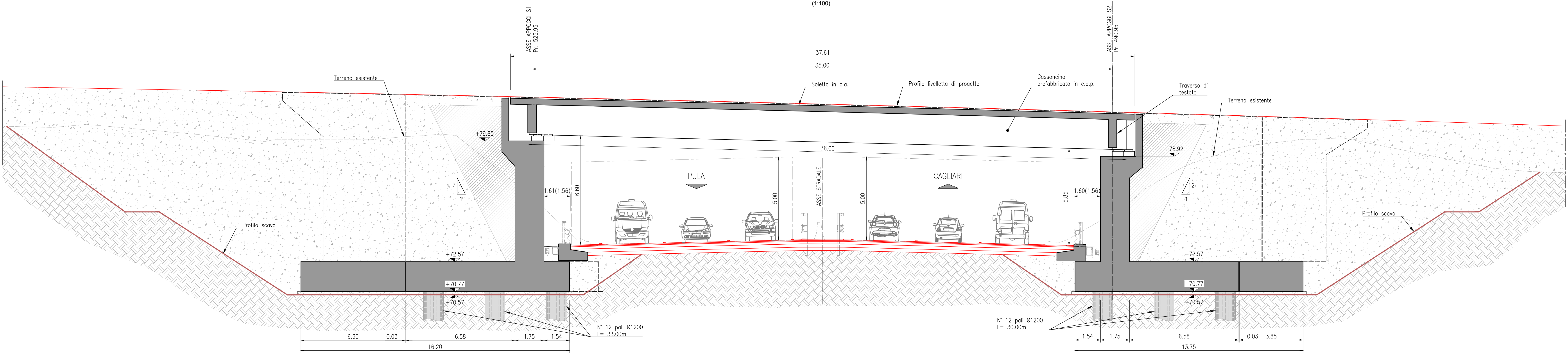
SEZIONE LONGITUDINALE IN ASSE STRADA (1:100)
