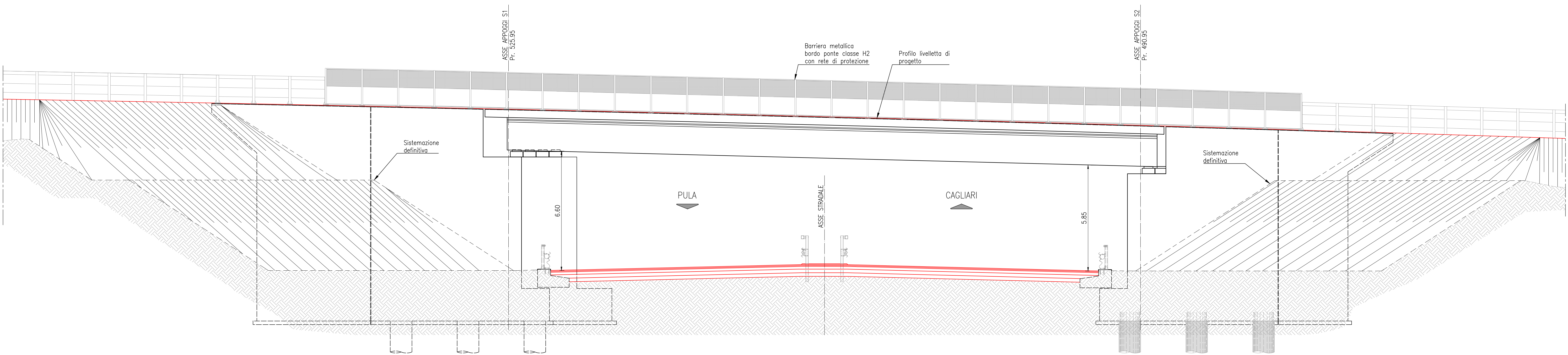
PROSPETTO SUD (1:100)
