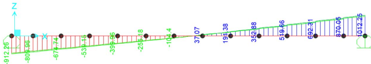
Figura 40 – Taglio Fase 3 – Inviluppo Combinazione SLV
