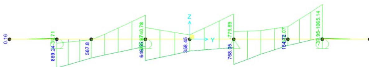
Figura 41 – Momento flettente Traverso di testata – Inviluppo Combinazione SLU
