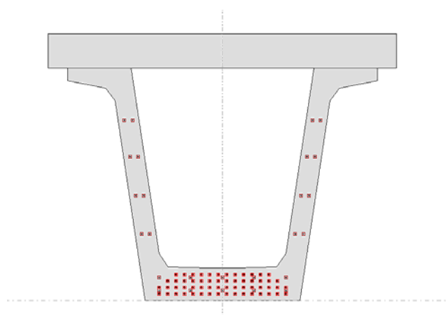
Figura 36 – Sezione di verifica - mezzzeria
