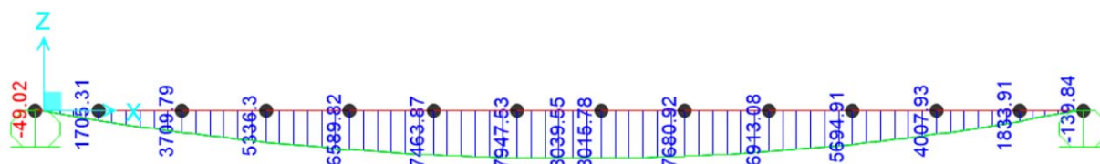
Figura 32 – Momento flettente Fase 3 – Combinazione SLE QP
