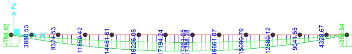
Figura 35 – Momento flettente Fase 3 – Involuppo Combinazione SLU
