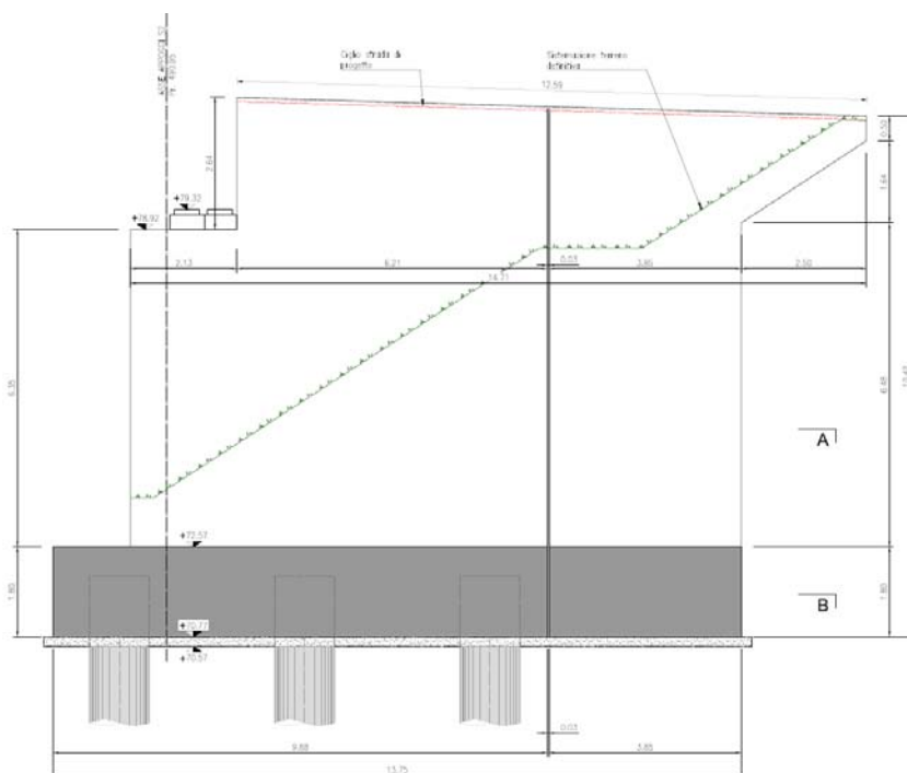
Figura 6 – Sezione trasversale e prospetto spalla S2
