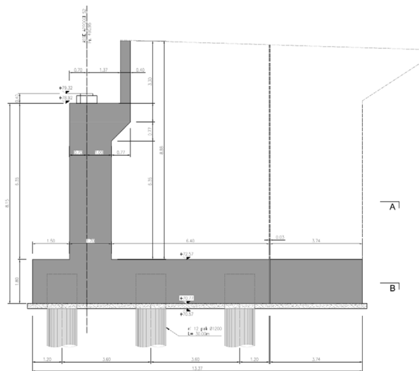
Figura 5 – Sezione trasversale e prospetto spalla S1
