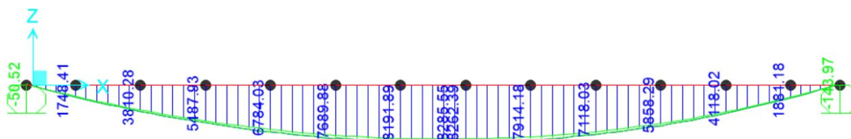
Figura 39 – Momento flettente Fase 3 – Inviluppo Combinazione SLV
