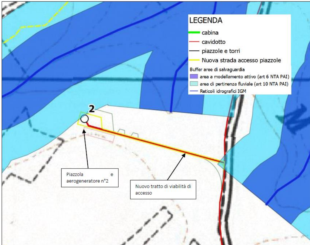
Figura 3-11: [WTG 2] Particolare della posizione dell'aerogeneratore, della piazzola e della nuova viabilità di accesso su stralcio cartografico IGM 1:25.000 rispetto alle fasce di salvaguardia di cui agli artt 6 e 10 delle NTA del PAI
