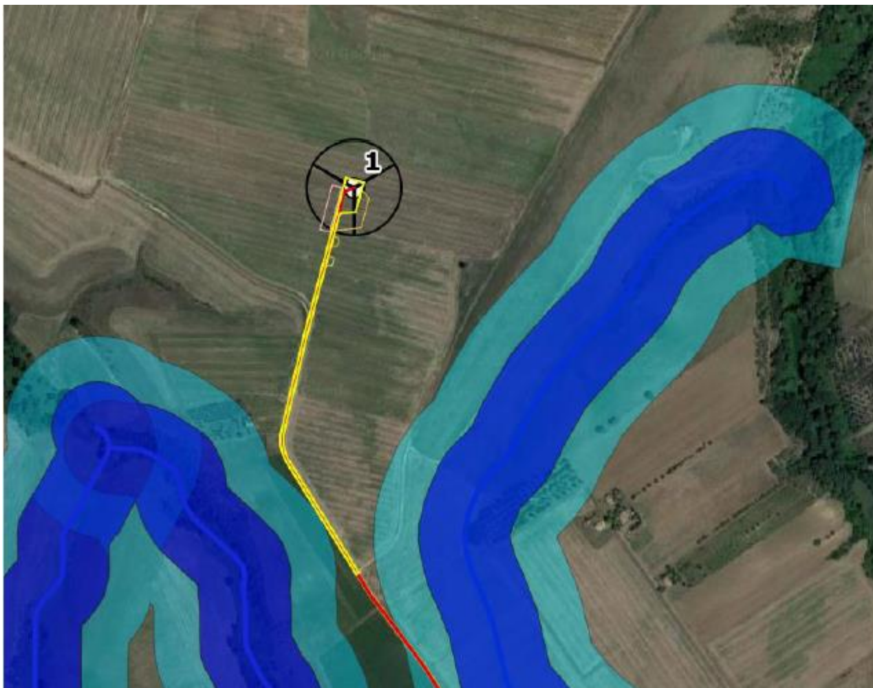
Figura 3-18: Verifica compatibilità torre WTG 1.
