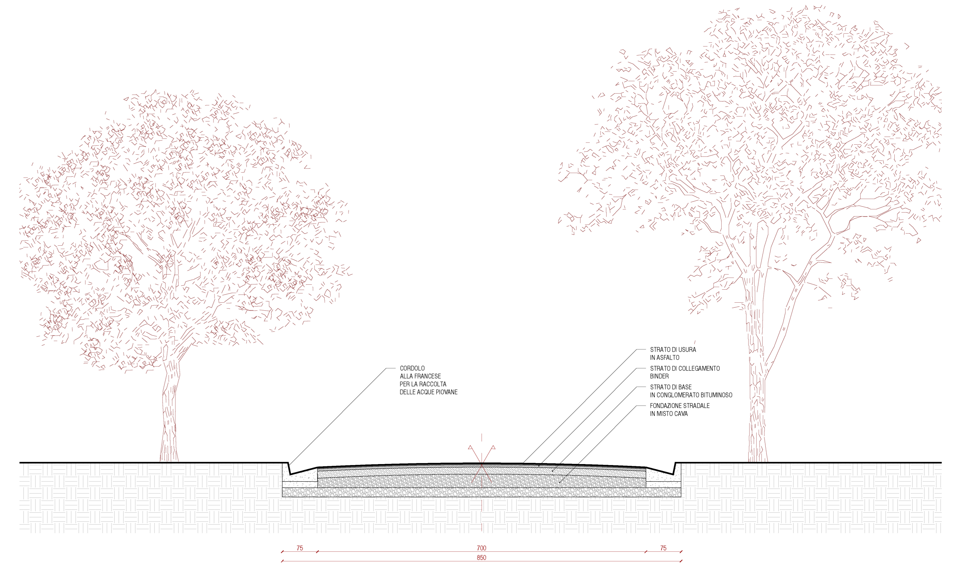
SEZIONE STRADALE | SCALA 1:50
