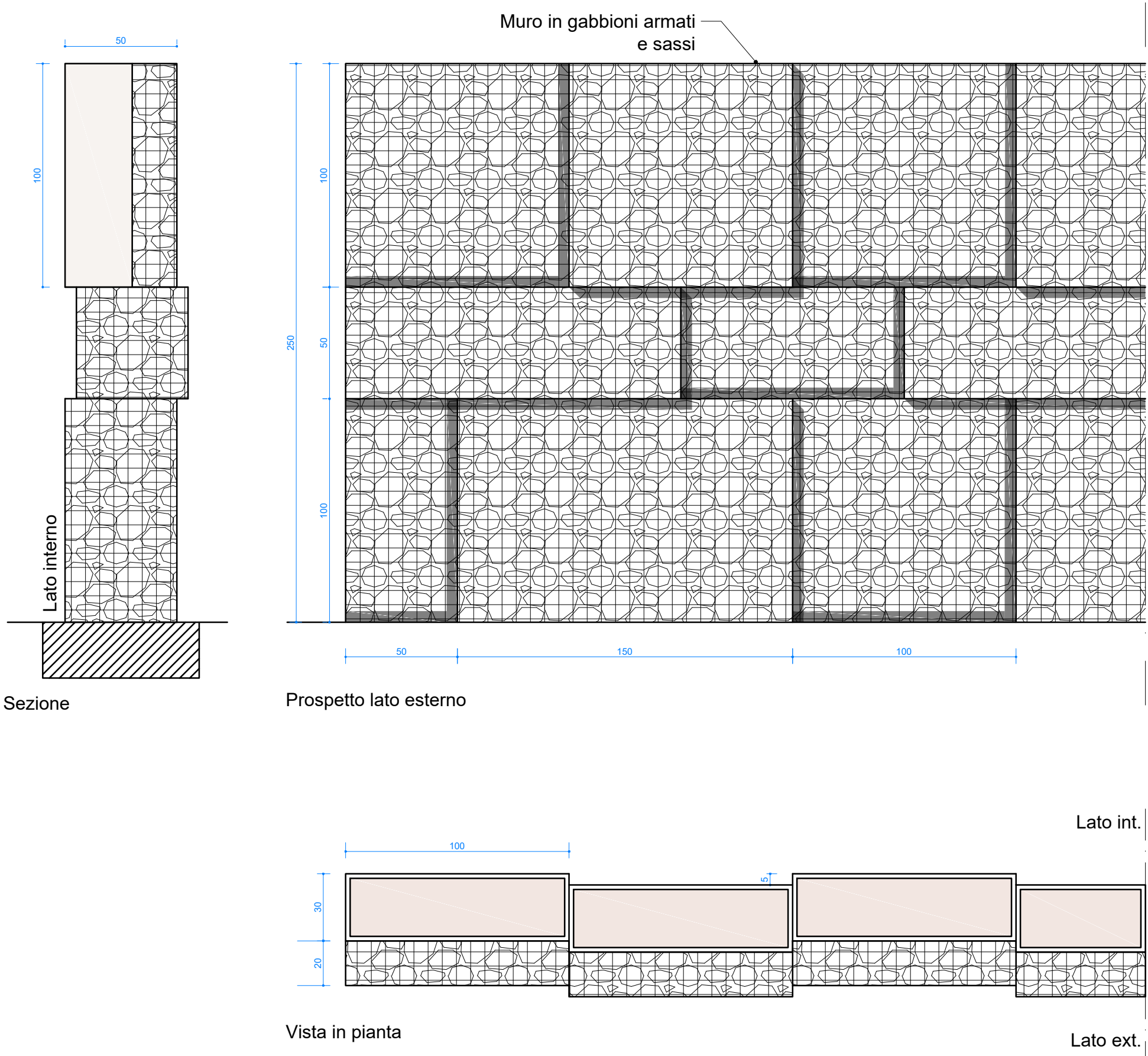
DETTAGLIO 1: RECINZIONE - SCALA 1:10
