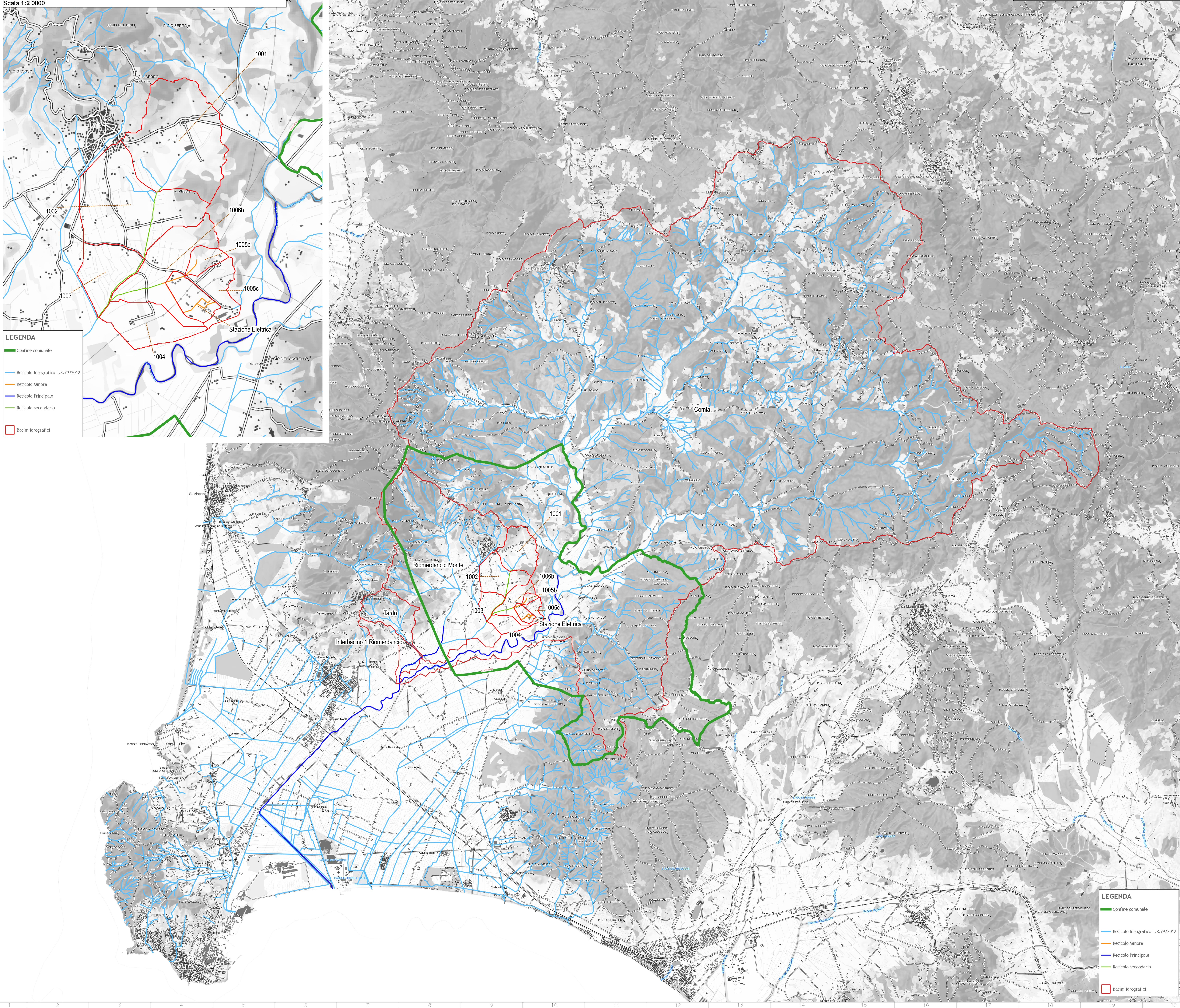
Planimetria dei bacini e del reticolo idrografico di studio Scala 1:50000
