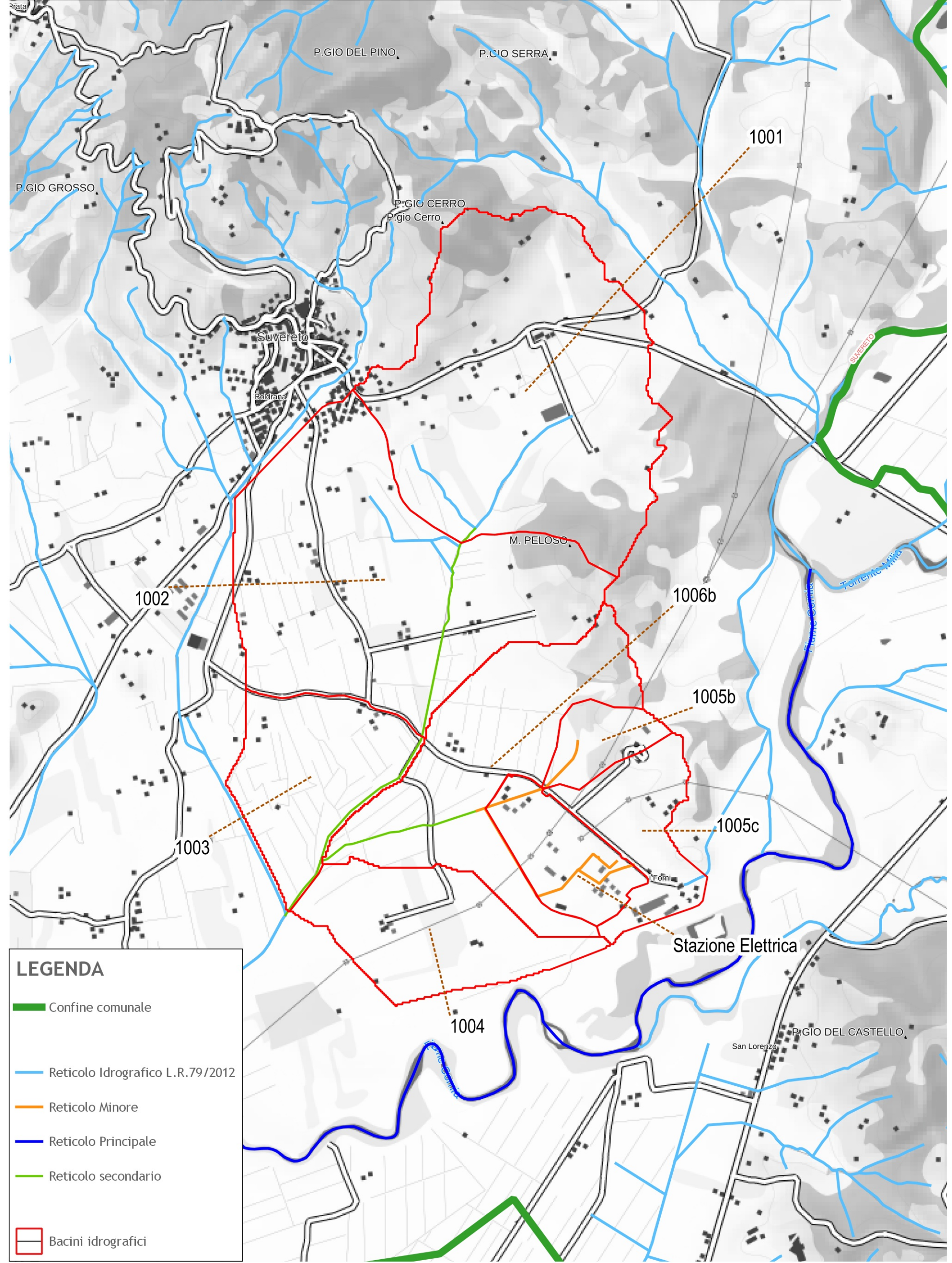
Planimetria dei bacini e del reticolo idrografico di studio - dettaglio reticolo secondario e minore Scala 1:2 0000
