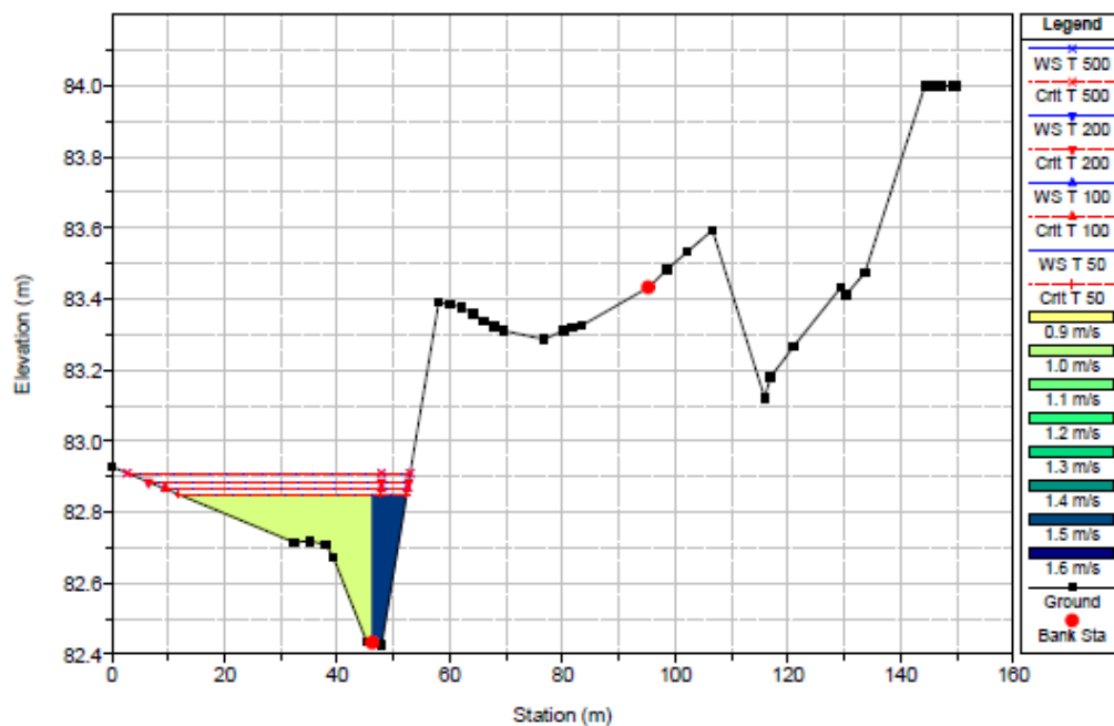
BACINO MUZZEDDU - Tronco Mz2 - sez.1150 - Estratto dall'elaborato R.B - Allegati alla Relazione di compatibilità idraulica
