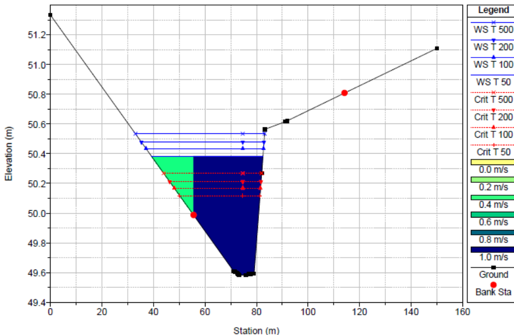
BACINO MUZZEDDU - Tronco Mz5 - sez.1400 - Estratto dall'elaborato R.B - Allegati alla Relazione di compatibilità idraulica
