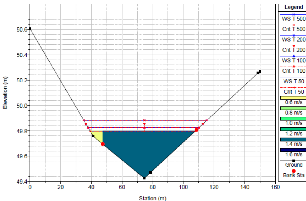
BACINO MUZZEDDU - Tronco Mz5 - sez.1350 - Estratto dall'elaborato R.B - Allegati alla Relazione di compatibilità idraulica
