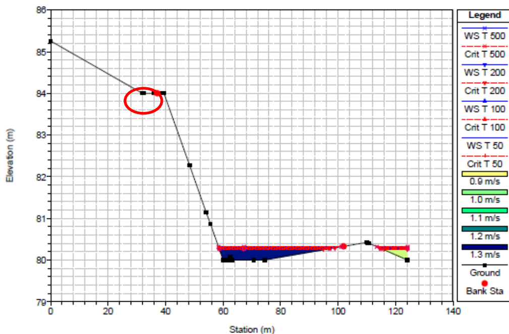
BACINO MUZZEDDU - Tronco Mz3 - sez.1100 - Estratto dall'elaborato R.B - Allegati alla Relazione di compatibilità idraulica
