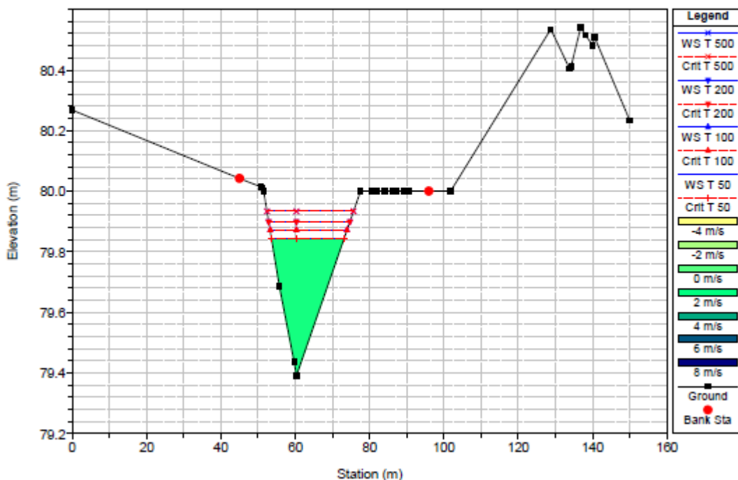
BACINO MUZZEDDU - Tronco Mz2 - sez.1100 - Estratto dall'elaborato R.B - Allegati alla Relazione di compatibilità idraulica
