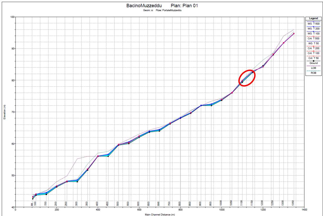
BACINO MUZZEDDU - Tronco Mz2 - Estratto dall'elaborato R.B - Allegati alla Relazione di compatibilità idraulica
