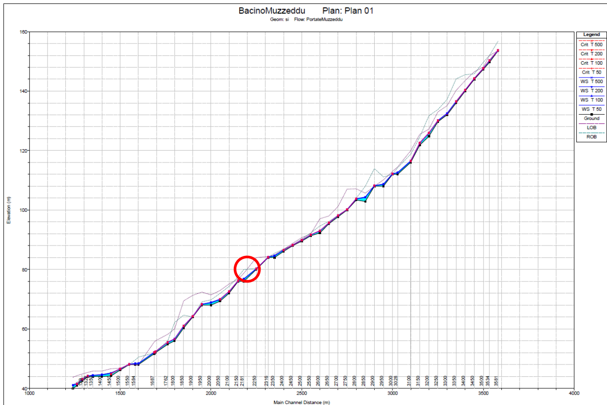
BACINO MUZZEDDU - Tronco Mz3 - Estratto dall'elaborato R.B - Allegati alla Relazione di compatibilità idraulica
