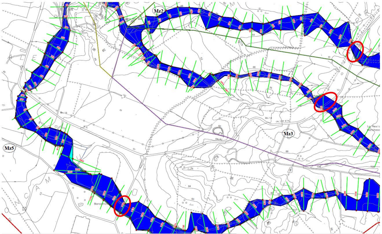
Estratto della Carta R.07 - Bacino Muzzeddu con individuazione dei tronchi interessati dalle intersezioni
