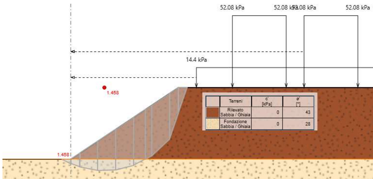
Condizione statica
