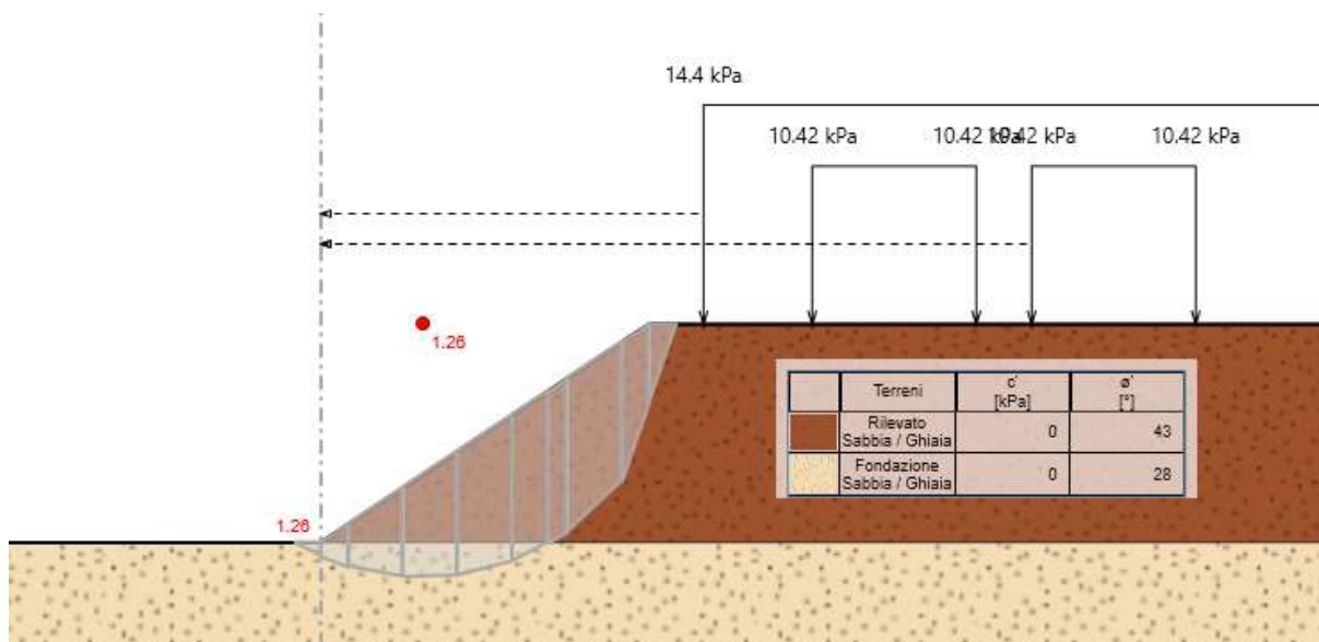
Condizione sismica
