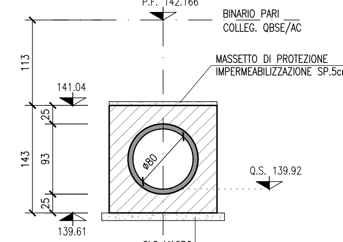
SEZIONE 6-6 SCALA 1:50
