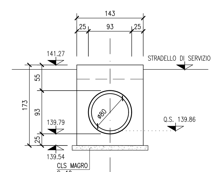
SEZIONE 4-4 SCALA 1:50
