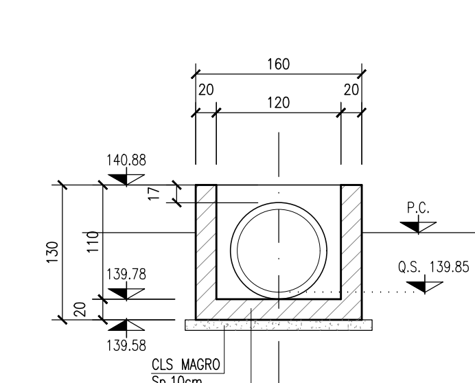
SEZIONE 5-5 SCALA 1:50
