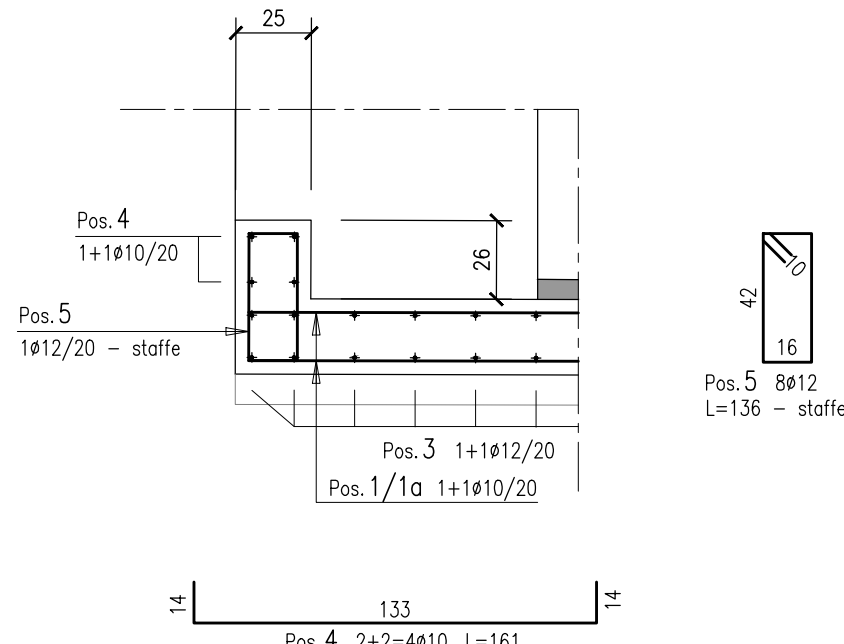
PART. "A" - ARMATURA IMBOCCO LATO L.S. SCALA 1:25
