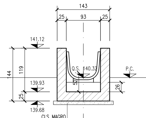
SEZIONE 4-4 SCALA 1:50
