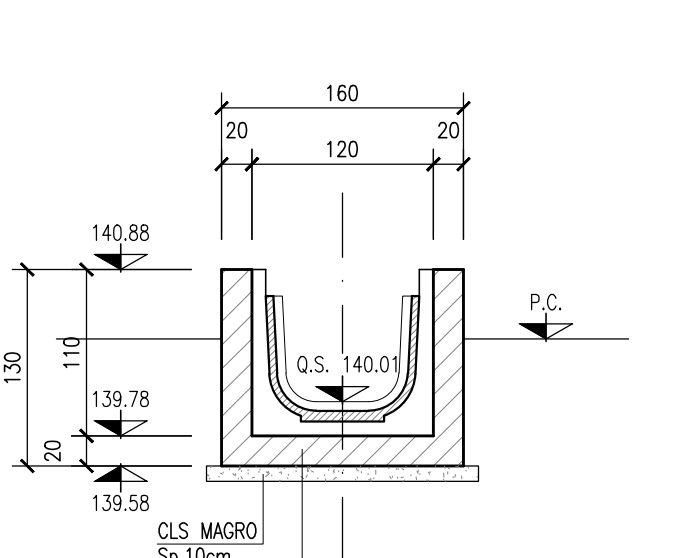
SEZIONE 6-6 SCALA 1:50
