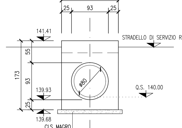
SEZIONE 5-5 SCALA 1:50
