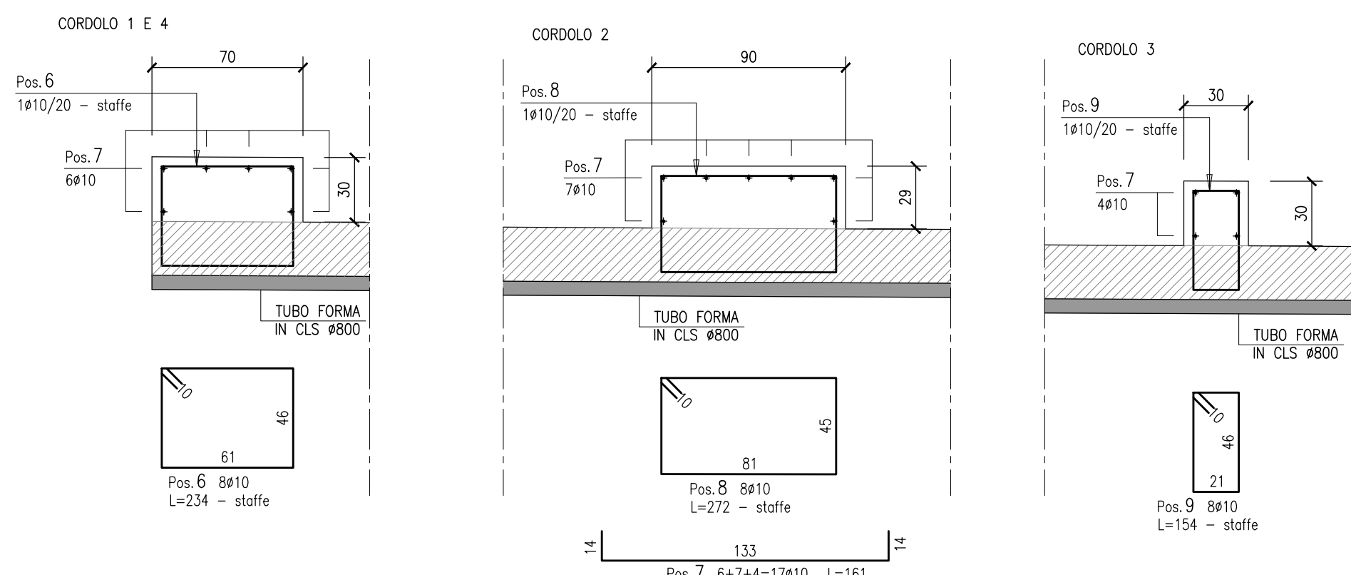
ARMATURA RIVESTIMENTO TUBO SCALA 1:25
