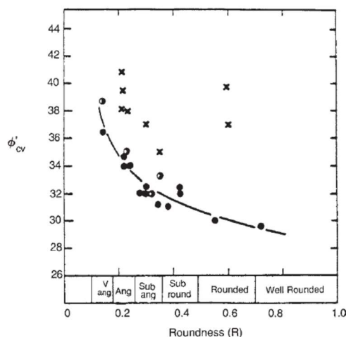
Figura 10-1 : valori indicativi di \phi'_{cv} , Youd (1972) (sinistra), Bolton (1986) (destra)
