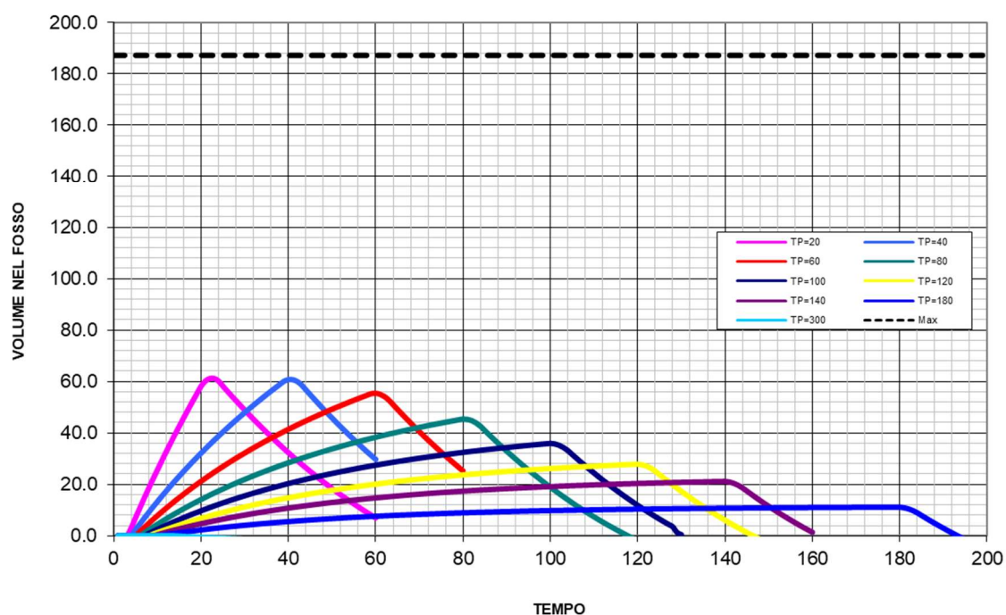
CURVE DEI VOLUMI INVASATI CON DIVERSE DURATE DI PIOGGIA
