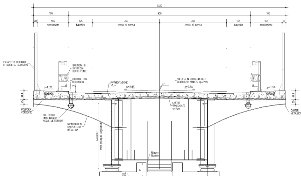
Figura 1 – Sezione trasversale impalcato
