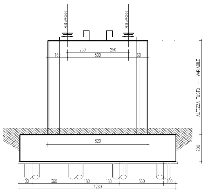
Figura 2 - Vista frontale pila
