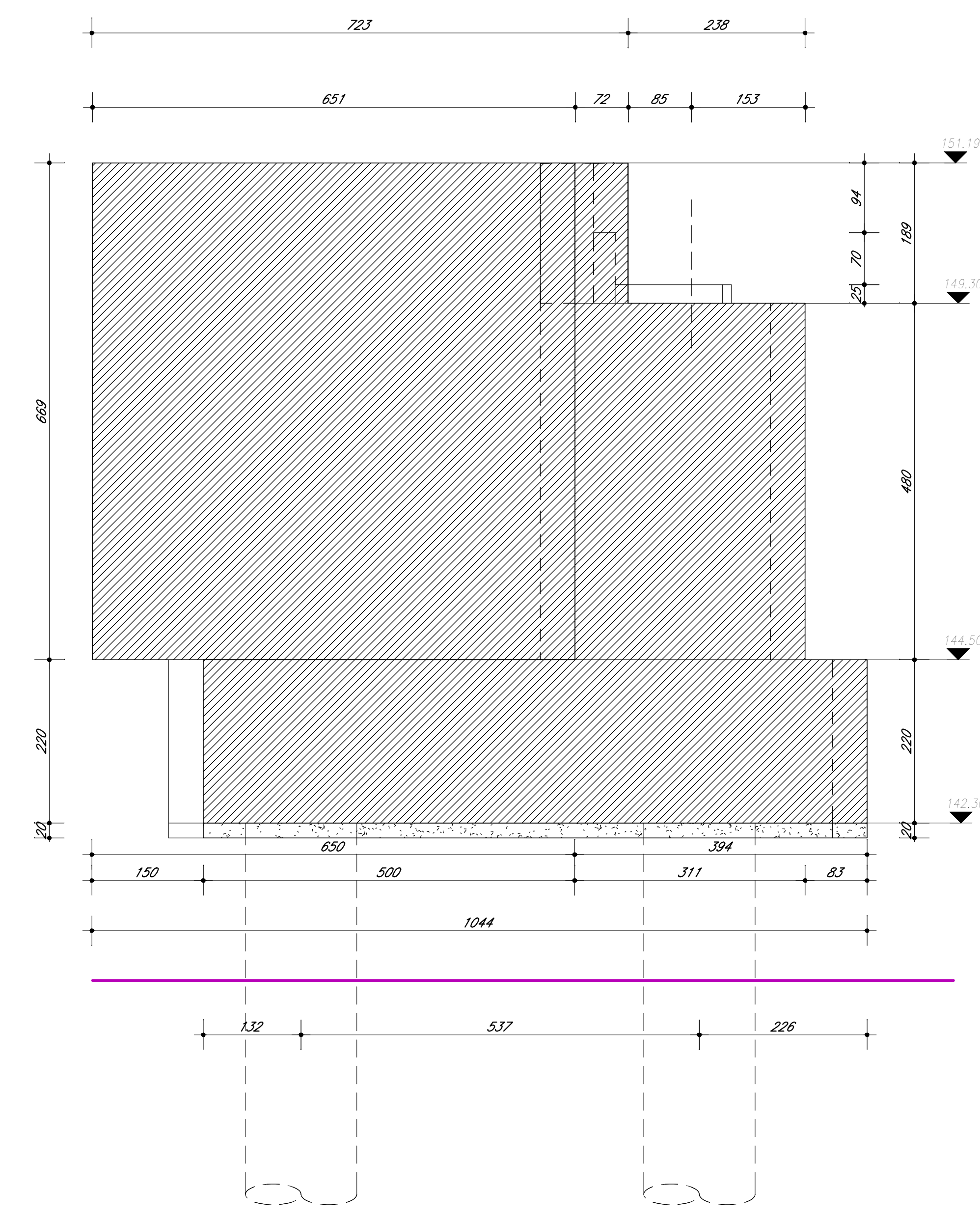
9 SpalloA - Prospetto lato 1 : 50
