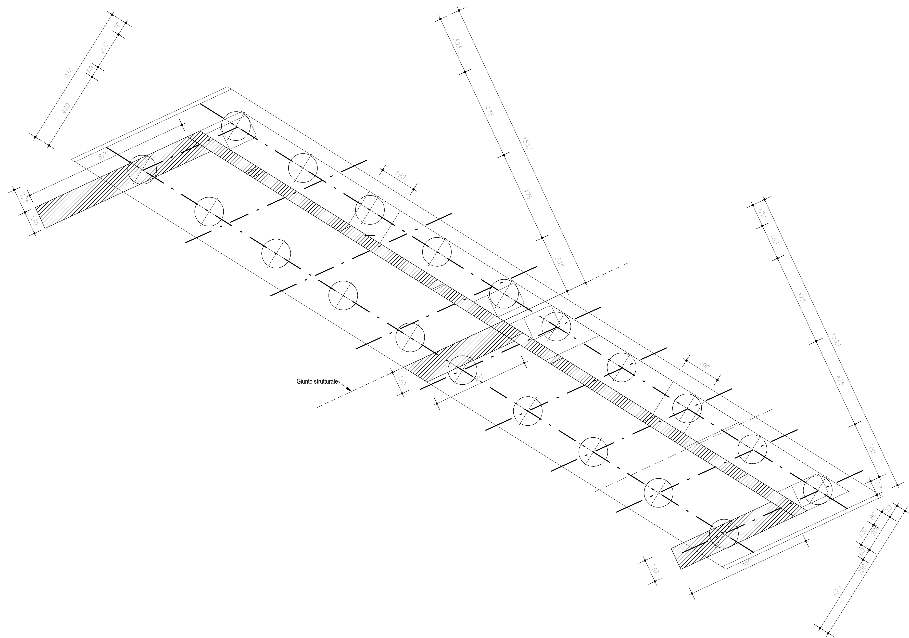
2 SpalloA - Vista dall'alto 1 : 100
