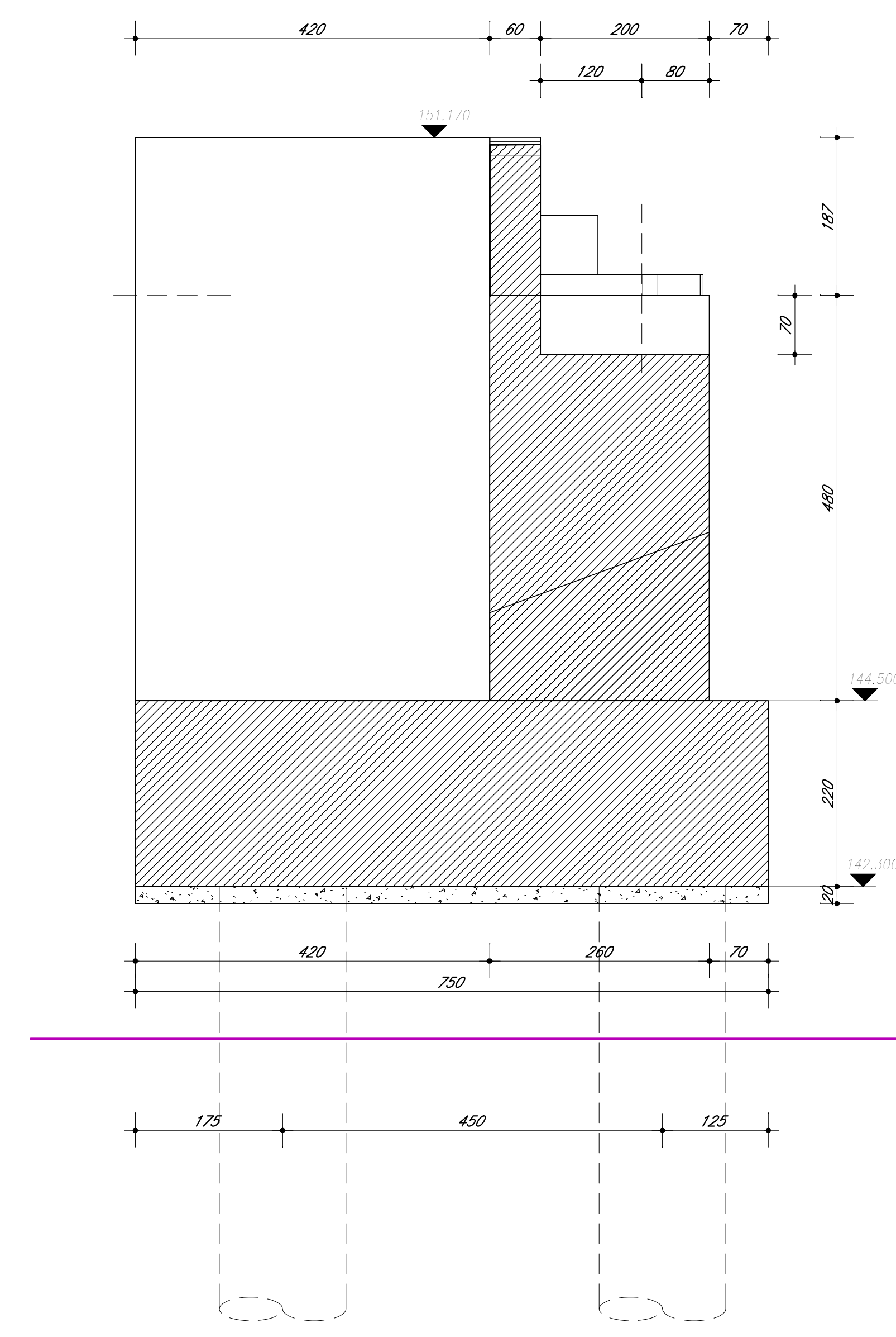
4 SpalloA - Sezione trasversale 1 : 50
