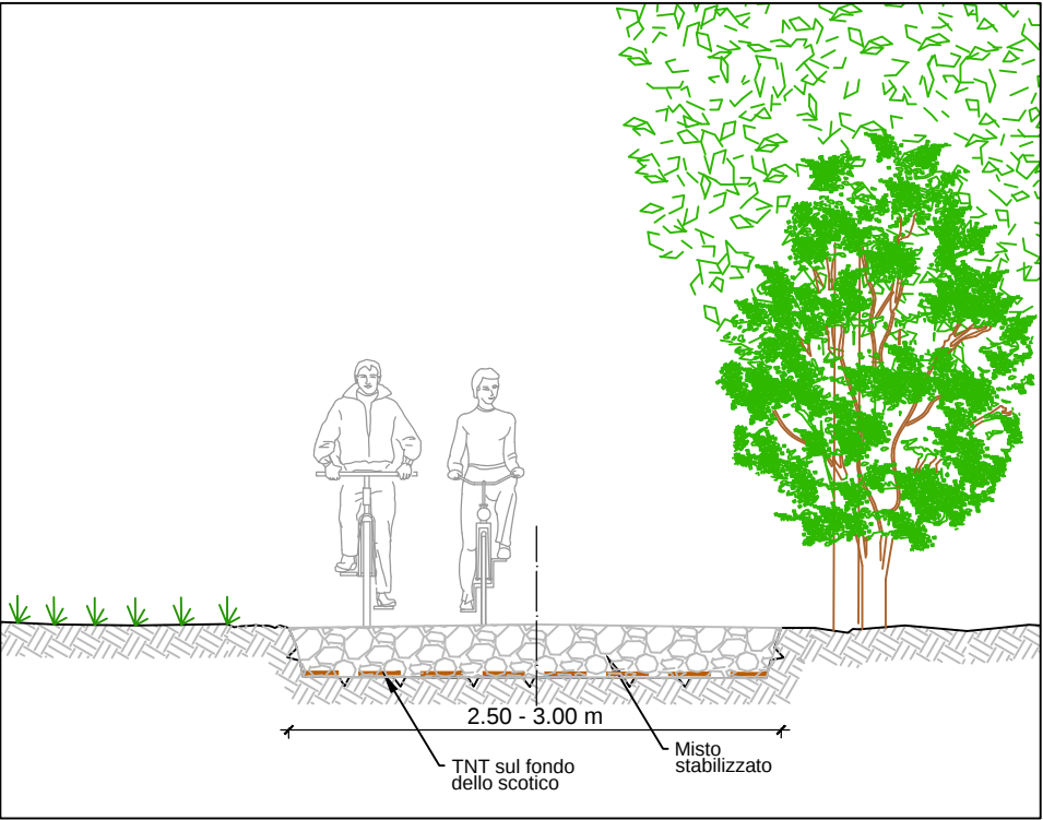
PISTA CICLABILE Sezione tipo scala 1:50
