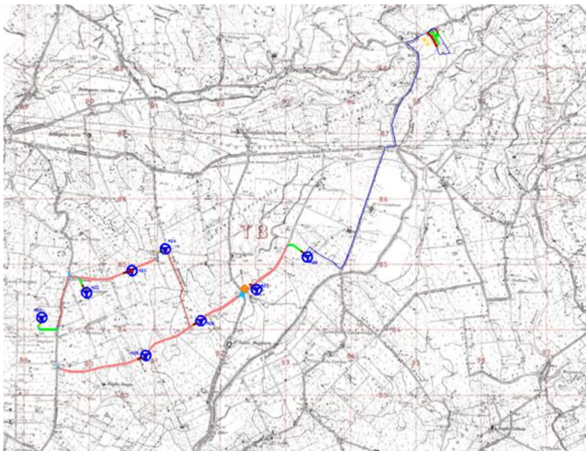
Layout del parco eolico su IGM
