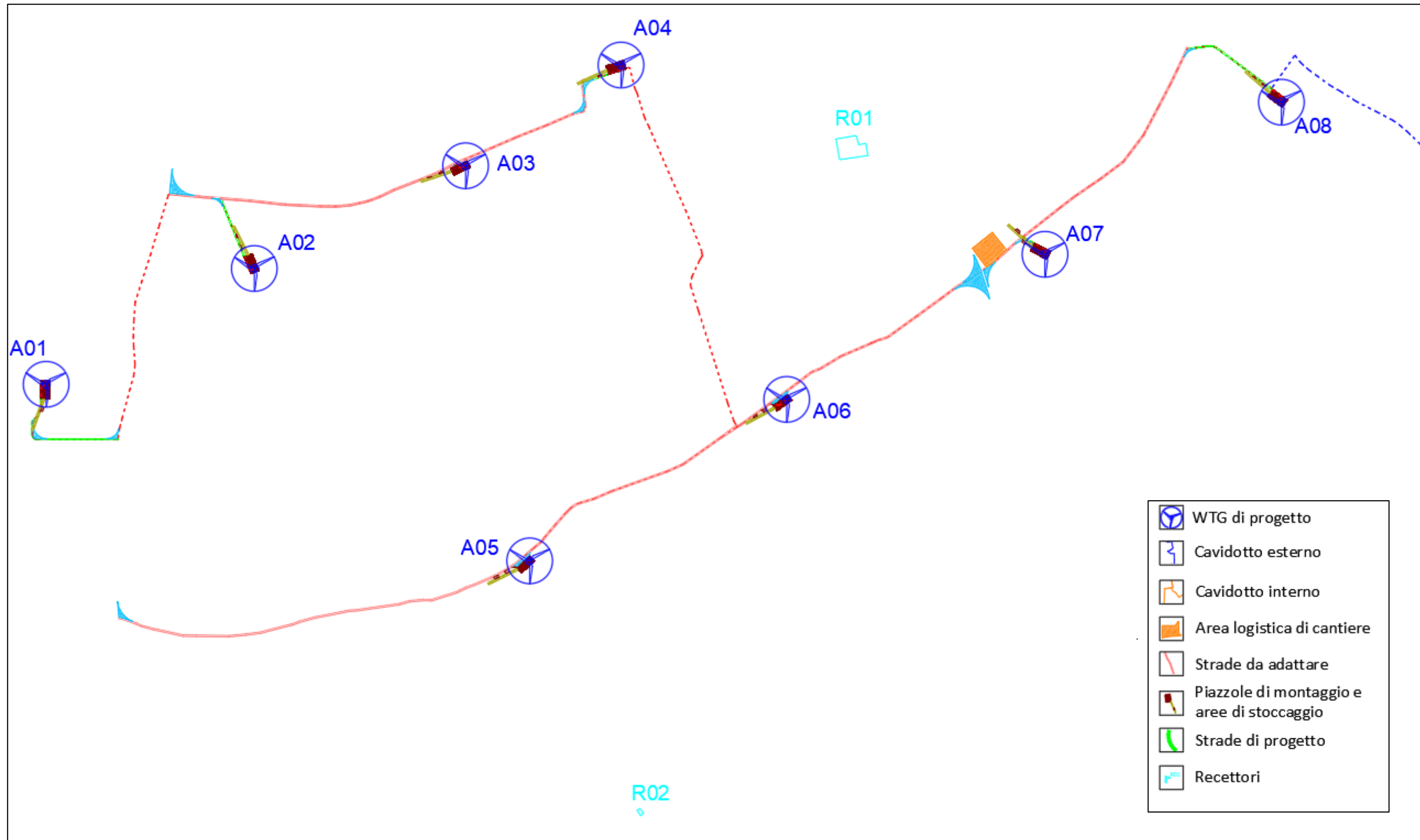
Figura 3: Inquadramento della viabilità di cantiere e delle aree di lavoro fisse e mobili.
