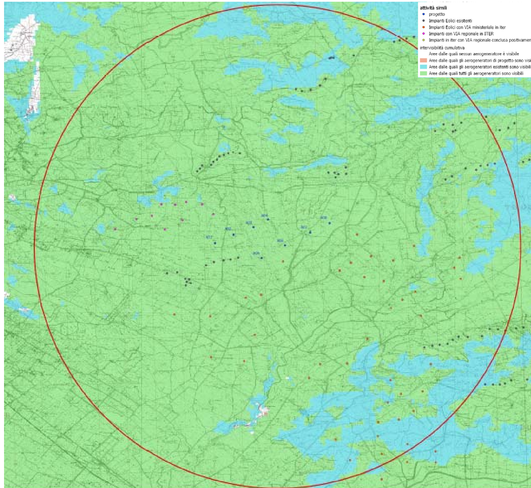
Figura 18: Mappa di intervisibilità cumulativa. Le aree da cui risulterebbe visibile il solo impianto di progetto (in blu) risultano una piccola estensione delle aree da cui sono visibili cumulativamente anche gli aerogeneratori esistenti, autorizzati ed in iter di approvazione. Sono rappresentate in ciano le aree da cui risultano visibili solo le turbine esistenti, autorizzate ed in iter approvativo. Considerato che la restituzione dello studio di intervisibilità, essendo potenziale, non tiene conto degli ostacoli presenti sul territorio, si può asserire a maggior ragione che non si determina alcun incremento dell'impatto percettivo.
