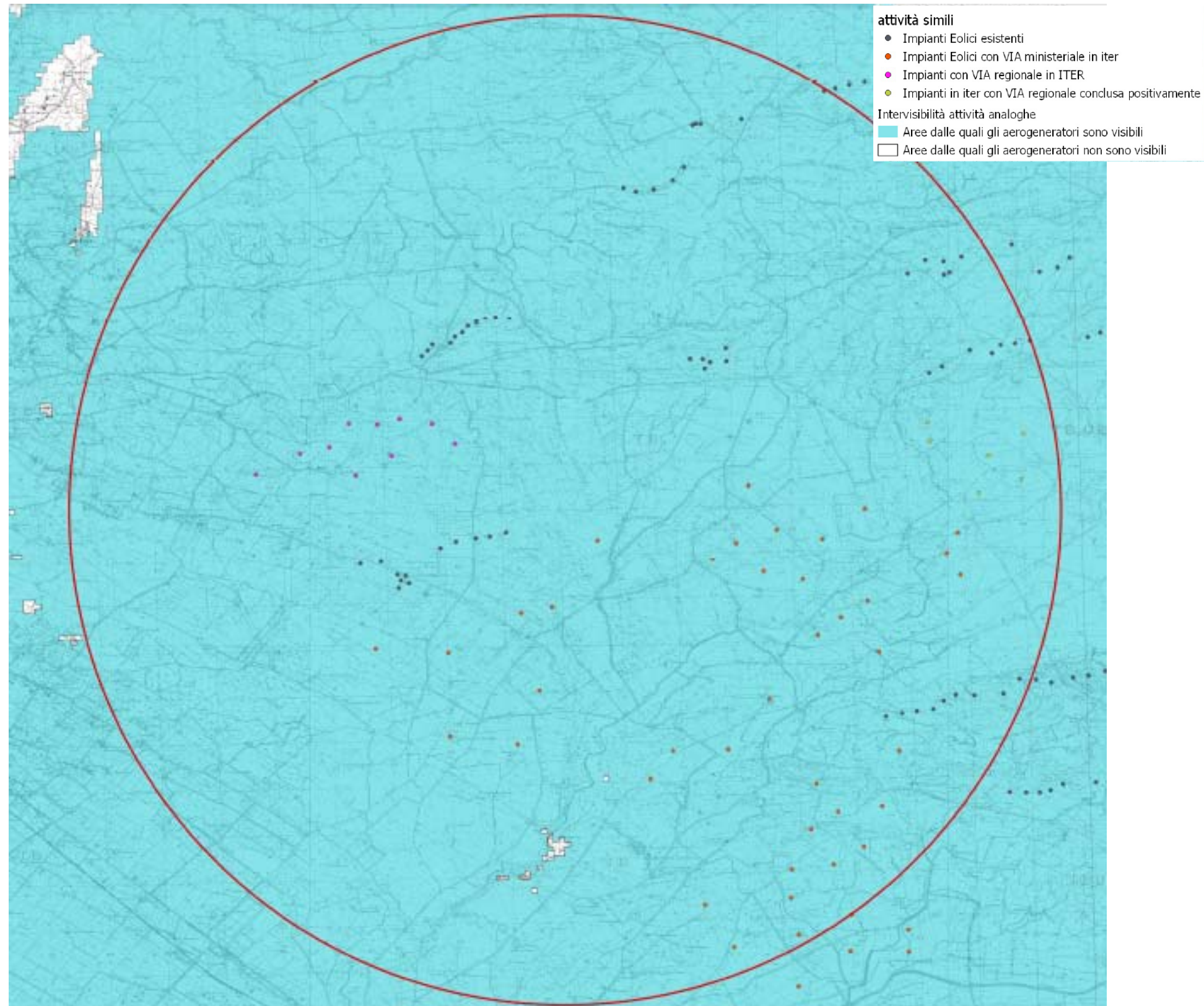
Figura 17: Mappa di intervisibilità riferita agli impianti esistenti, autorizzati, ed in iter autorizzativi. In ciano le porzioni di territorio da cui sono teoricamente visibili gli impianti esistenti, autorizzati ed in iter autorizzativo ricompresi nell'areale, tenendo conto solo dell'orografia e non degli ostacoli presenti (alberature, fabbricati, ...).
