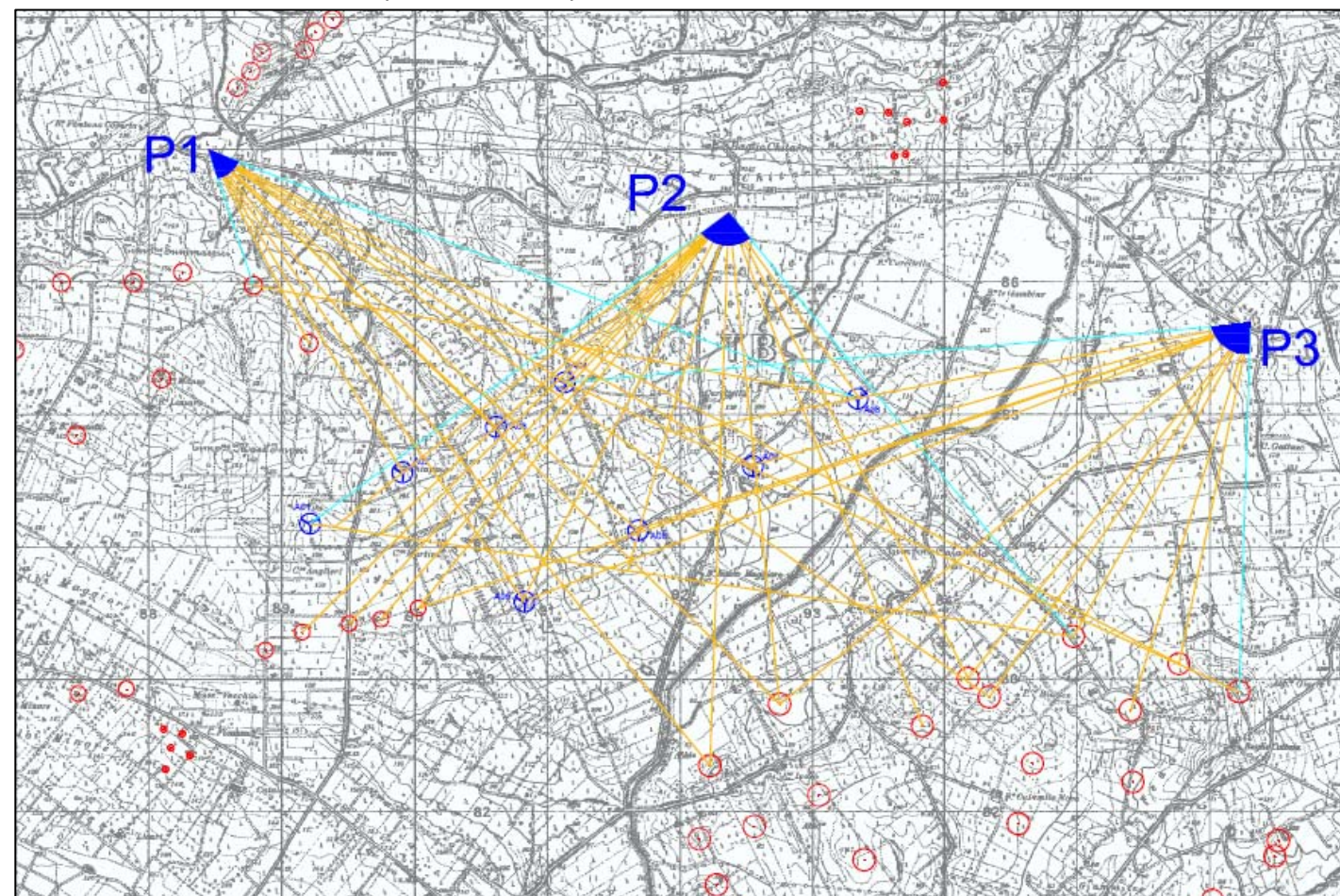
Figura 19: Punti di osservazione (in blu), campi visivi (in ciano) e linee di costruzione per il calcolo degli indici di affollamento (in giallo). In blu gli aerogeneratori di progetto, in rosso le turbine realizzate, autorizzate e in iter.
