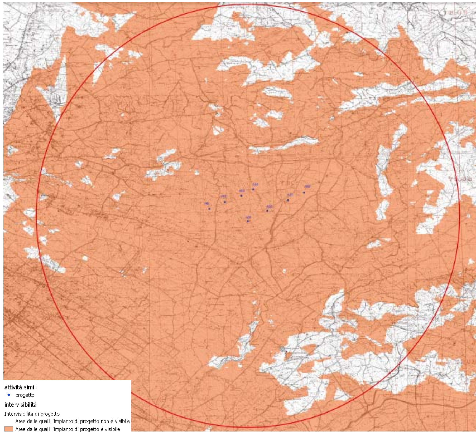
Figura 16: Mappa di intervisibilità di progetto. In arancione le porzioni di territorio da cui è teoricamente visibile l'impianto, tenendo conto solo dell'orografia e non degli ostacoli presenti (alberature, fabbricati, ...). Aerogeneratori di progetto in blu.
