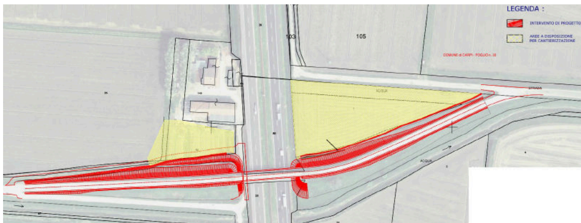
Figura 6: Planimetria dell'intervento con indicazione in rosso del limite dell'area di intervento e in giallo il perimetro all'interno del quale saranno ubicate le aree logistiche e di deposito delle (Fonte: Allegati alla Lista di controllo)
