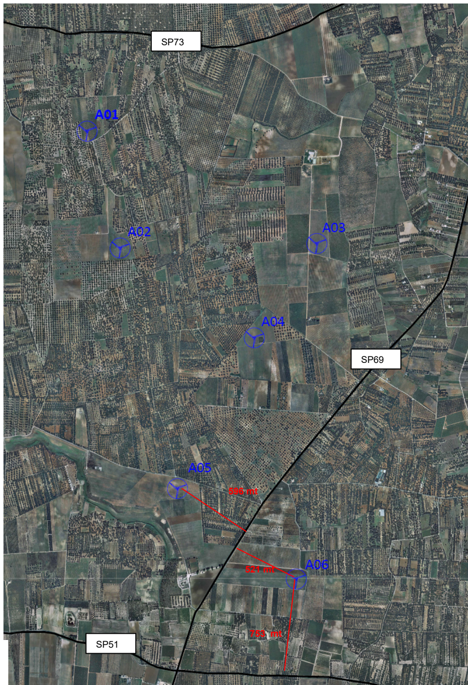
Figura 3: Distanze minime degli aerogeneratori dalle strade provinciali
