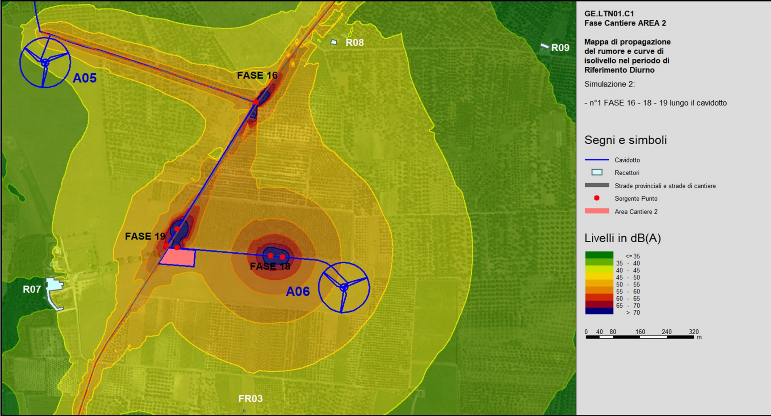
MAPPA DI PROPAGAZIONE DEL RUMORE - AREA 2, SIMULAZIONE 2
