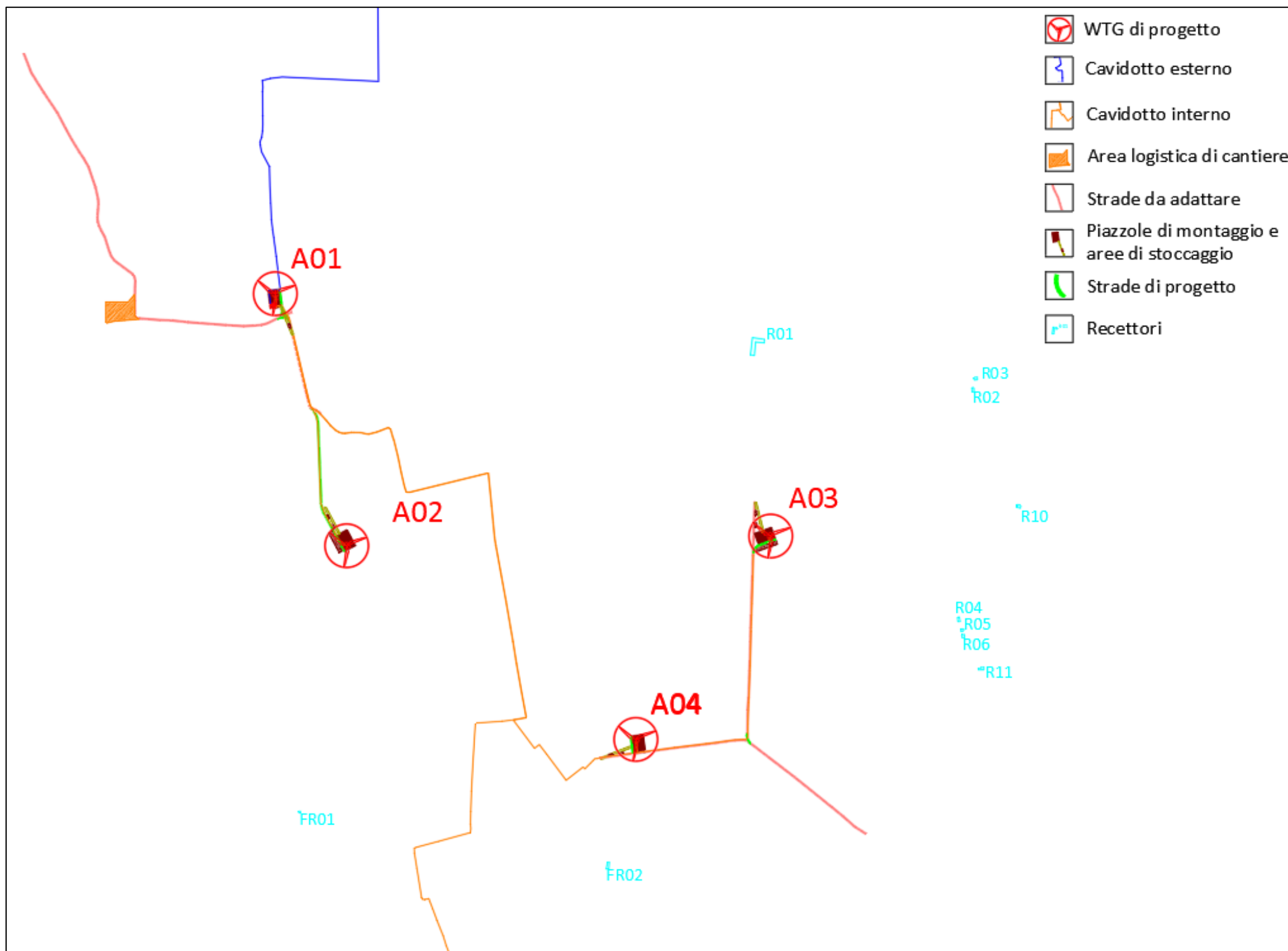
Figura 4: Inquadramento della viabilità di cantiere e delle aree di lavoro fisse e mobili relativo all'Area 1.
