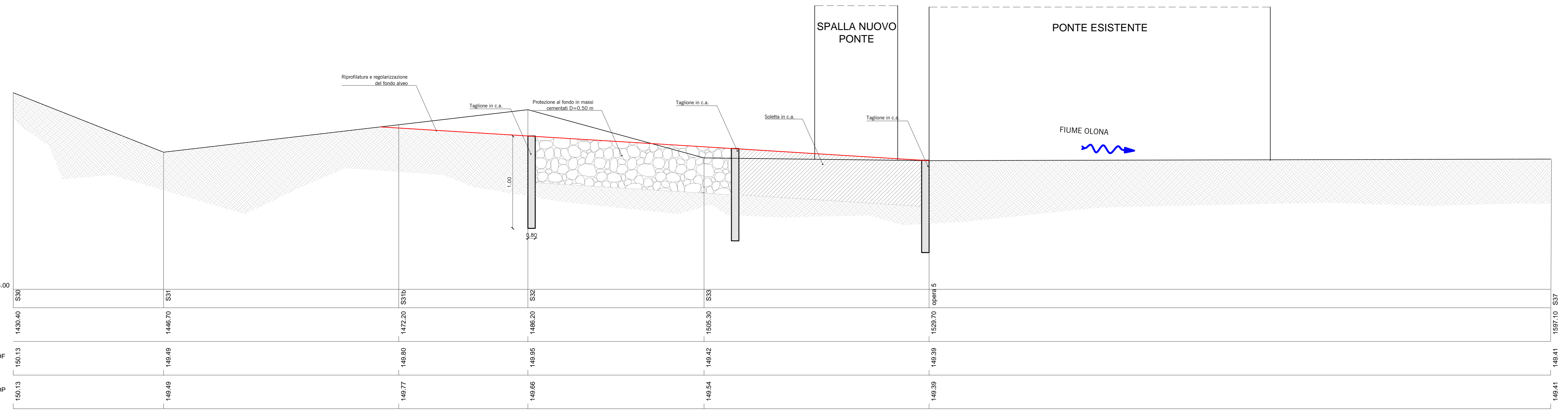
SISTEMAZIONE IDRAULICA DEL FONDO: PROFILO LONGITUDINALE
