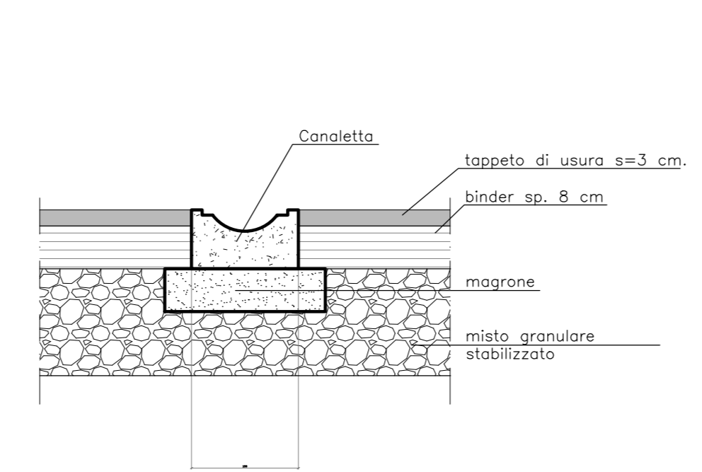
PART. CANALETTA CONTINUA 1:10
