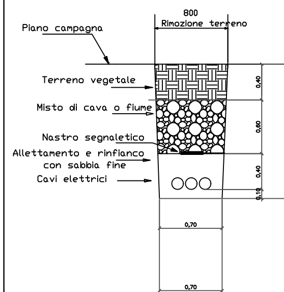
CAVIDOTTO 150 kV IN TERRENO NORMALE 1 TERNA
