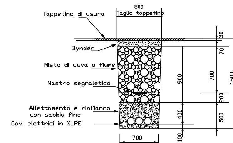
CAVIDOTTO 150 kV SOTTO SEDE STRADALE 1 TERNA
