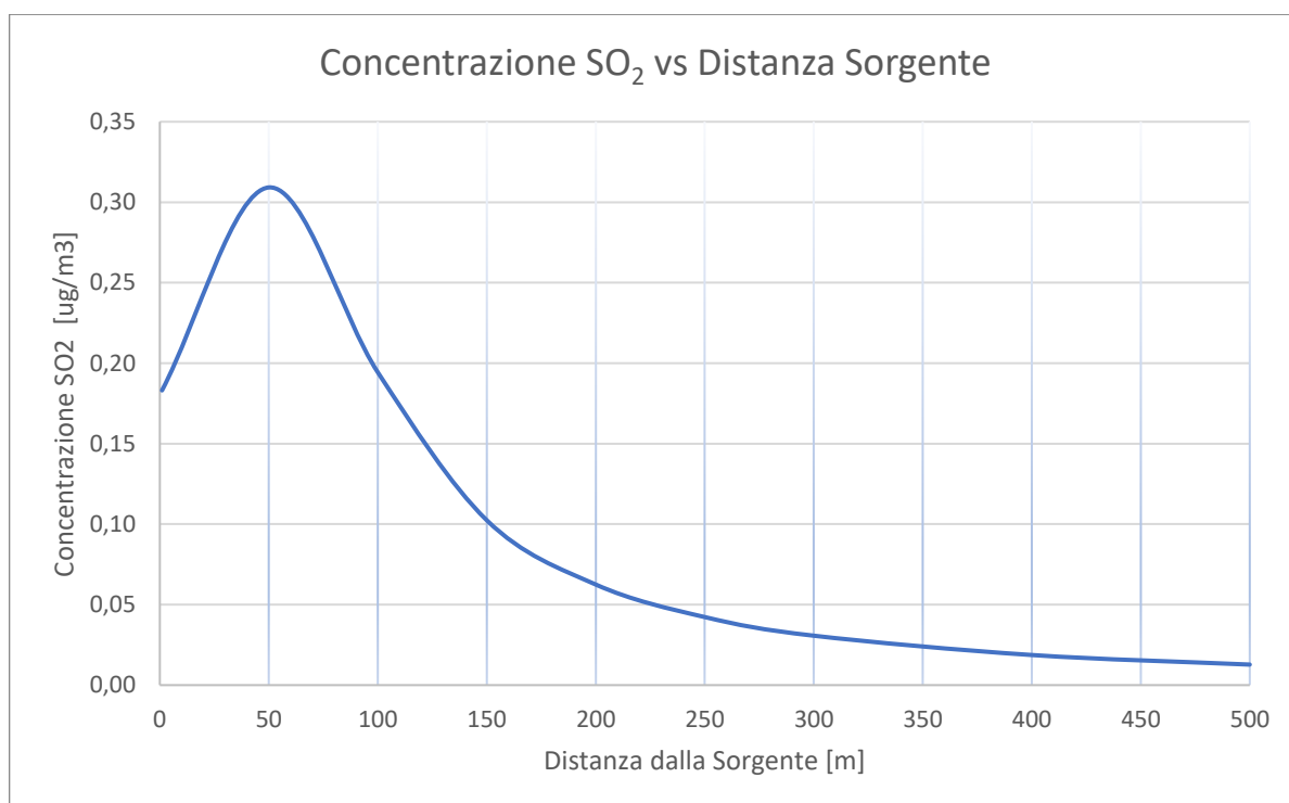
Figura 6-3 Concentrazione SO 2 vs Distanza dalla sorgente
