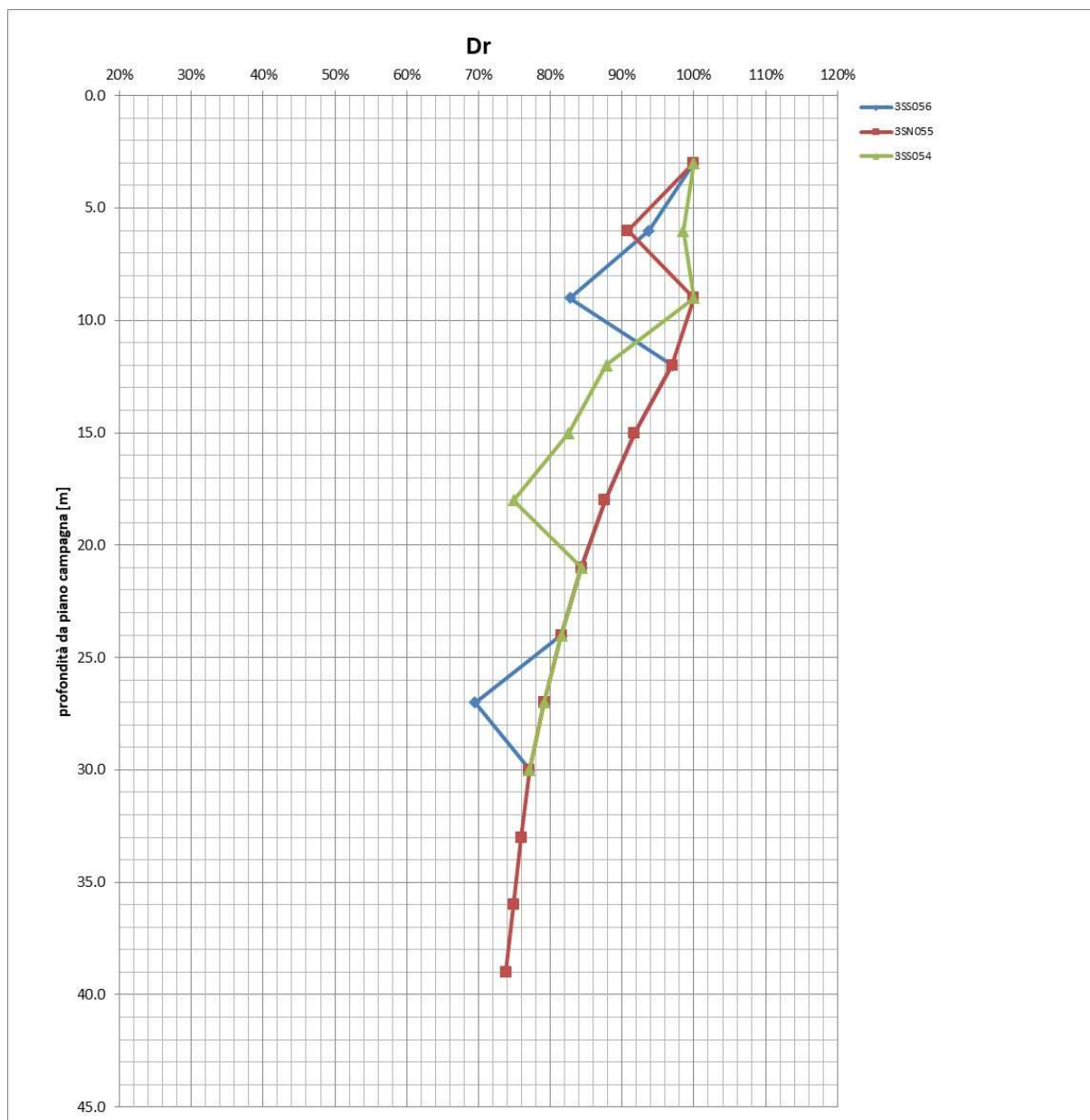
Figura 17-3: Andamento con la profondità della densità relativa ricavata dall'interpretazione dei risultati delle prove N_{SPT}
