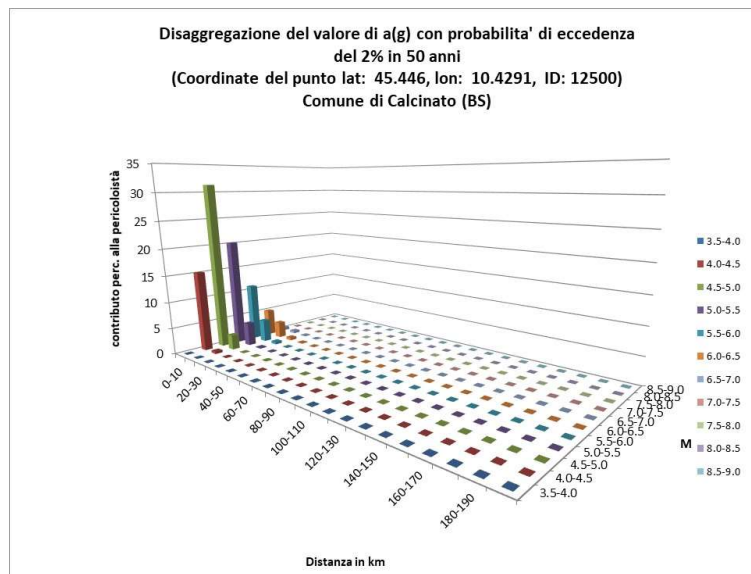
Figura 10-2: Contributi specifici magnitudo-distanza alla pericolosità sismica (Comune di Calcinato)
