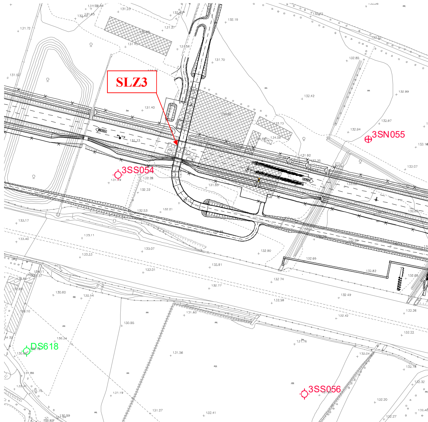
Figura 5-1 Stralcio planimetrico con sondaggi
