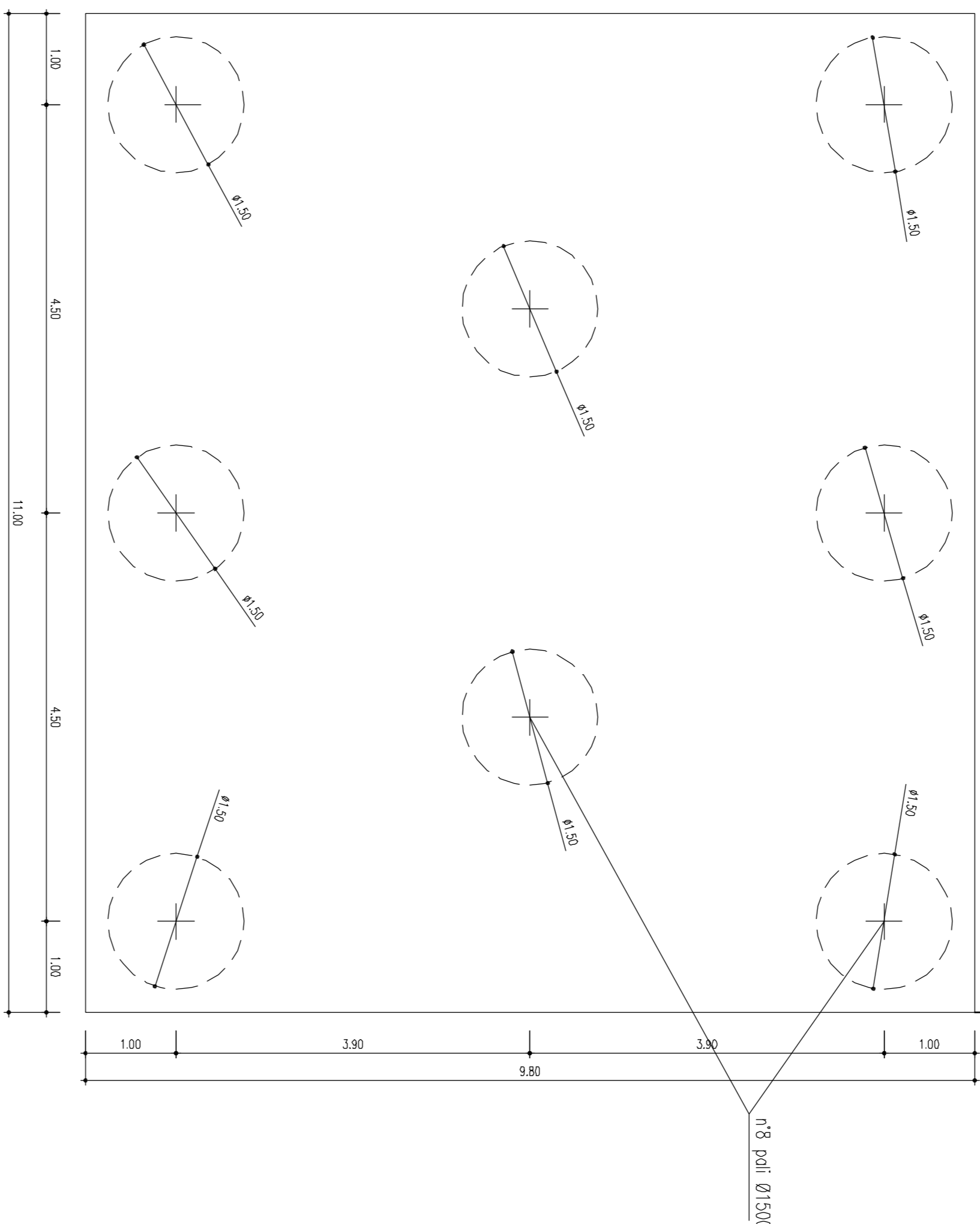
PIANTA FONDAZIONI
