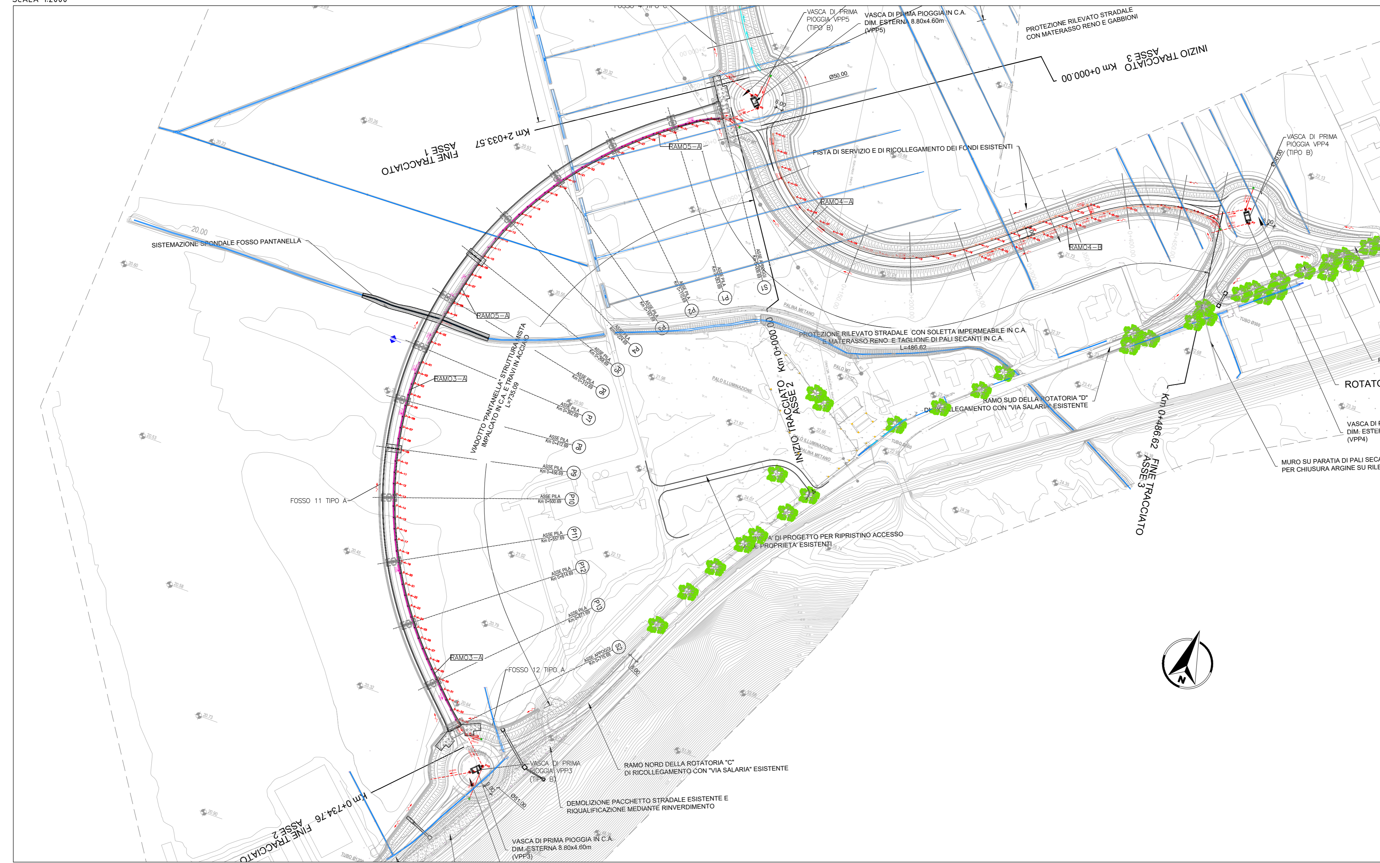
PLANIMETRIA ASSE 2 SCALA 1:2000
