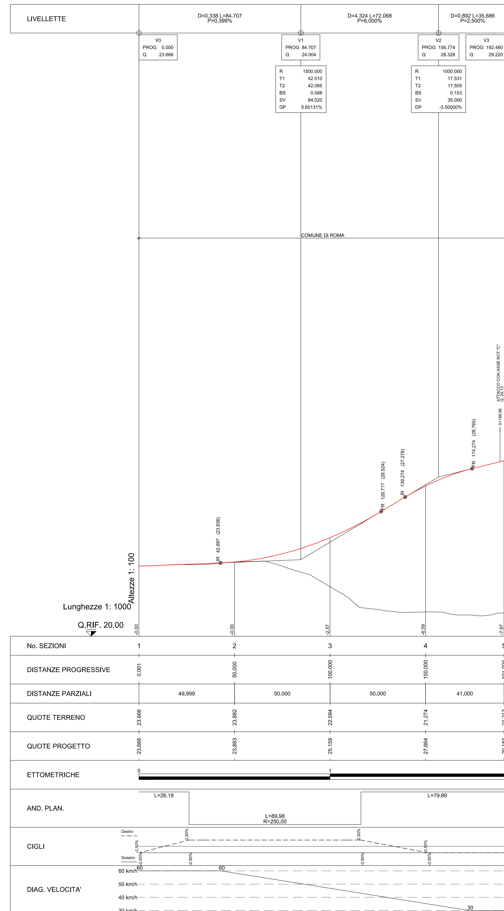
PROFILO LONGITUDINALE BRACCIO SUD
