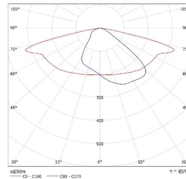
CURVA FOTOMETRICA
