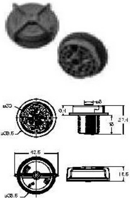
PARTICOLARE DISPOSITIVO PUNTO-PUNTO PER CORPO ILLUMINANTE
