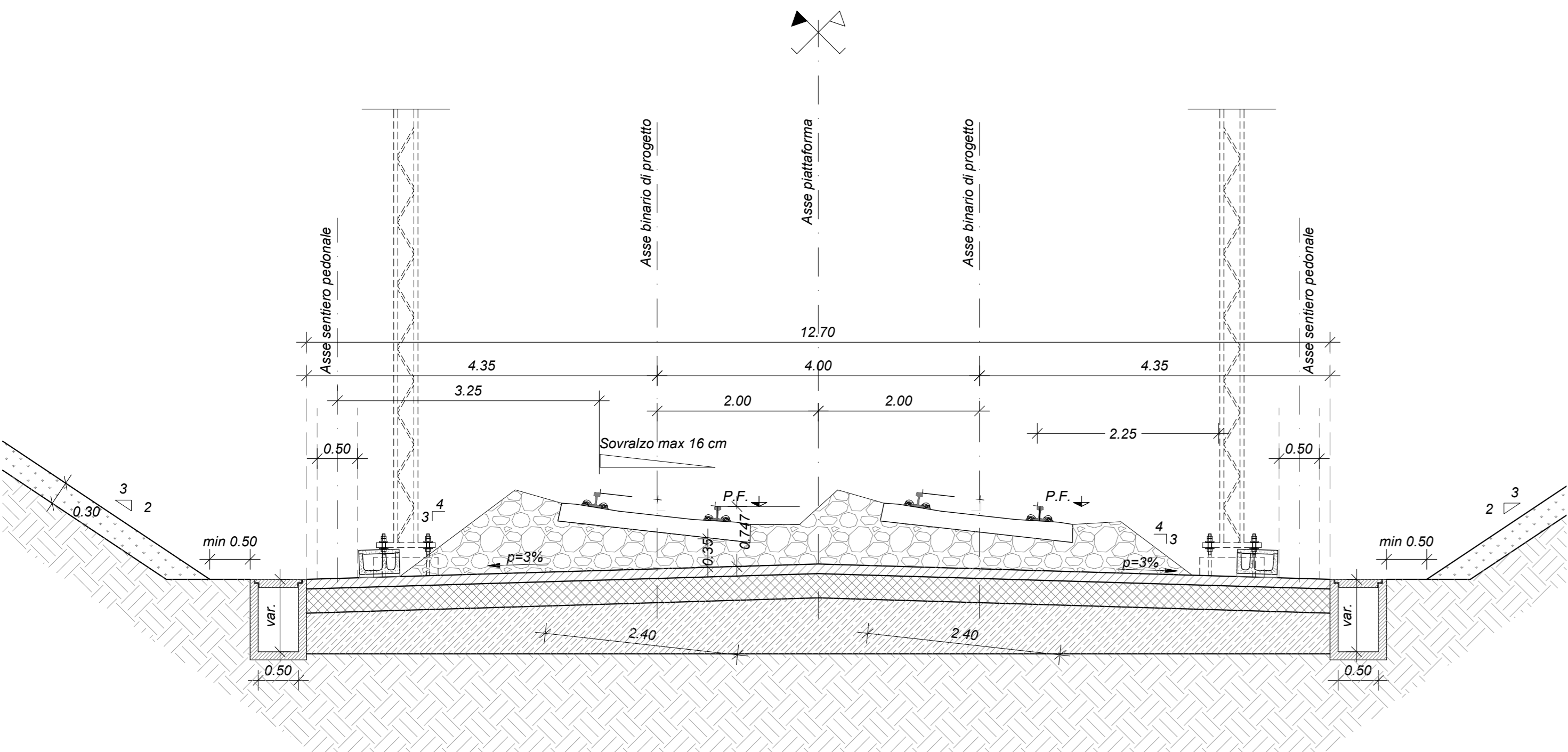
Sezione in curva
