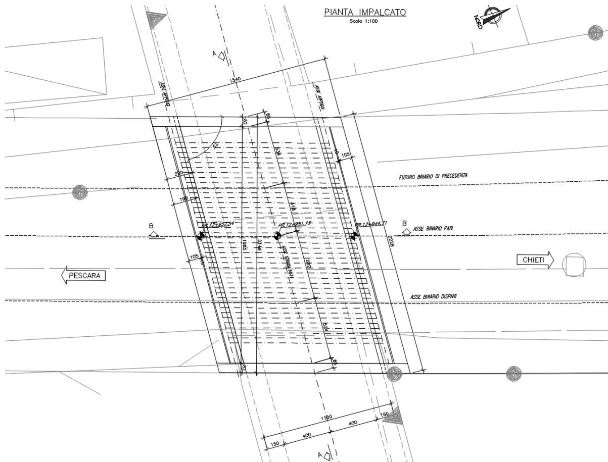
Figura 3: Pianta appoggi
