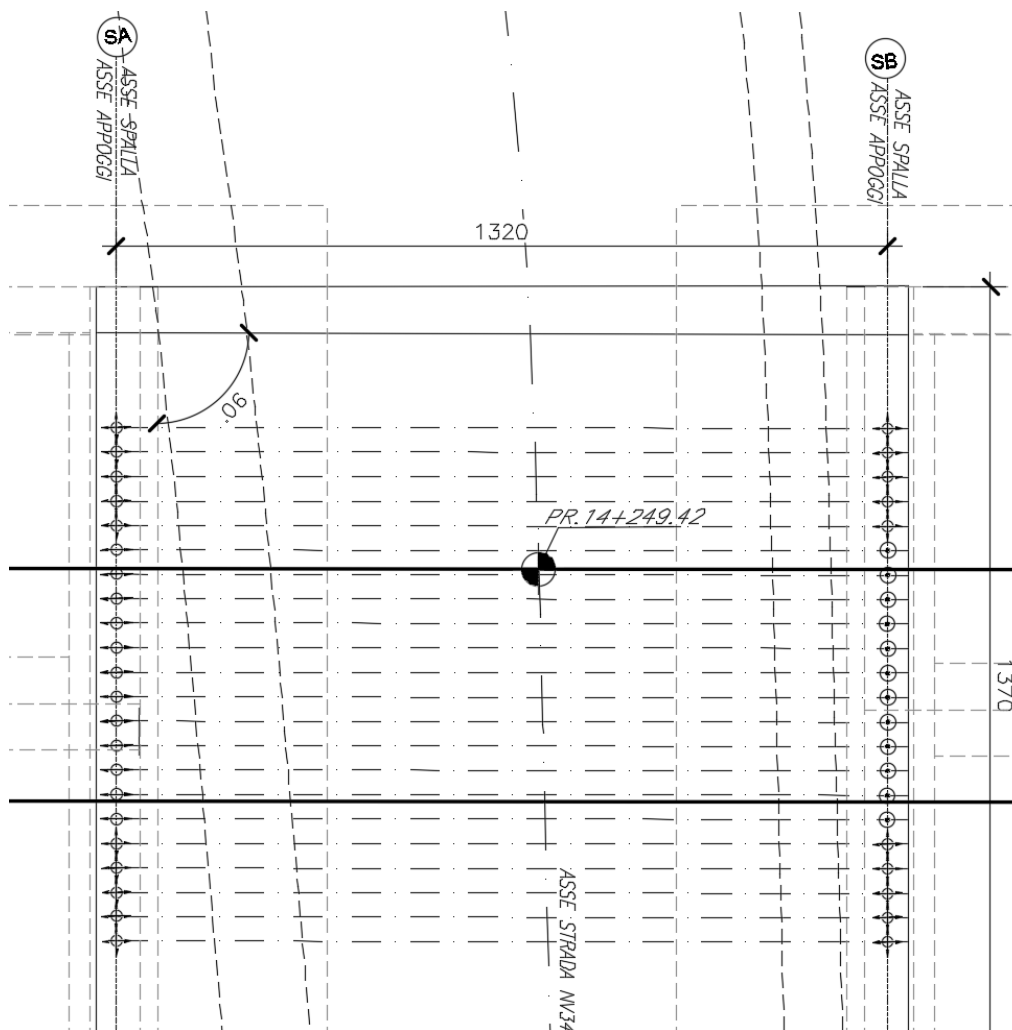
Figura 8: Pianta appoggi
