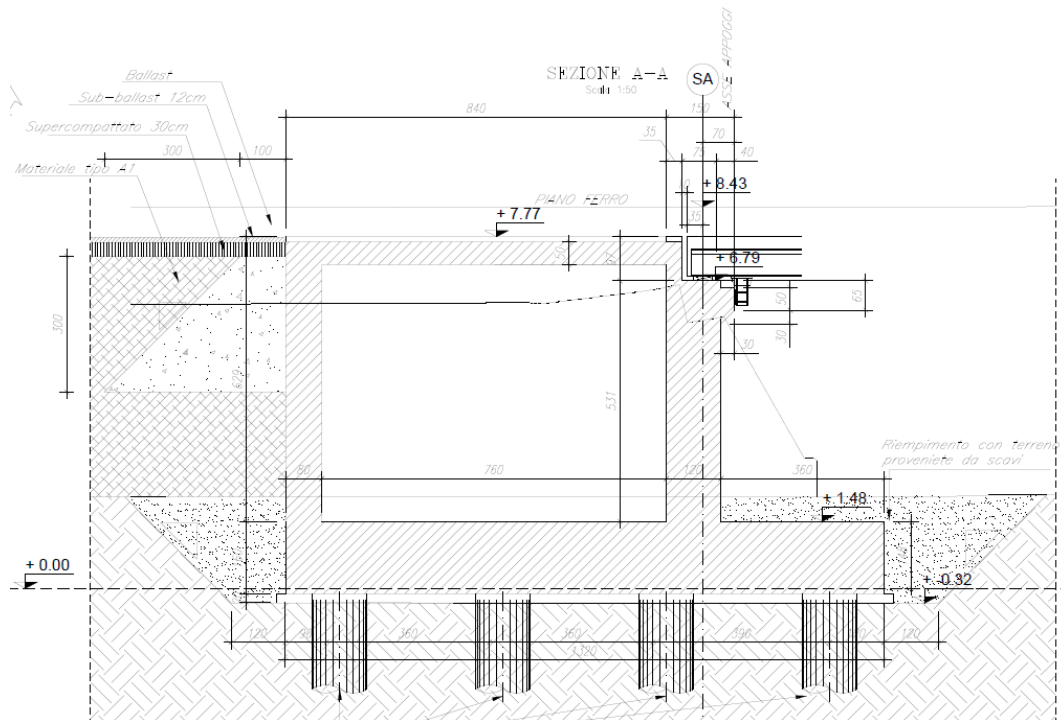
Figura 10 Sezione longitudinale (in asse tracciamento) della spalla
