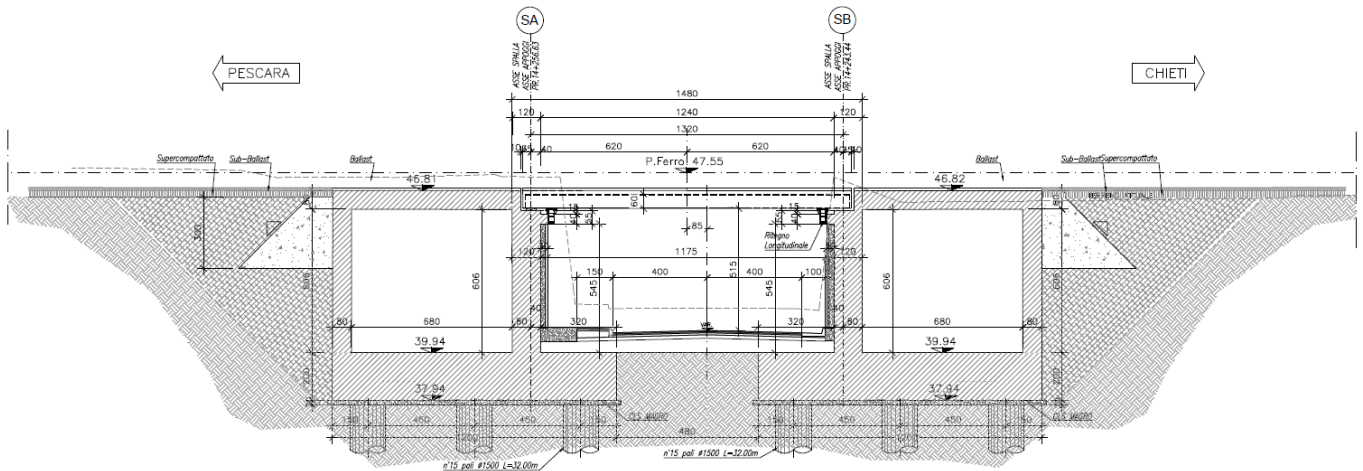
Figura 7: Sezione longitudinale dell'opera
