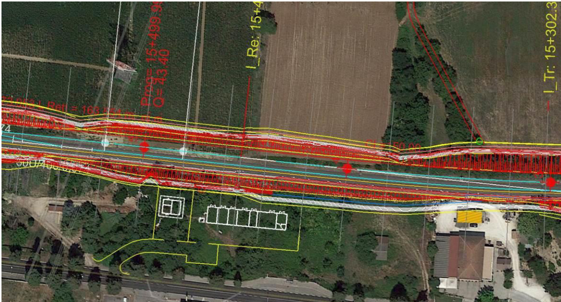
Figura 2-10: Piazzale tecnologico PT03
