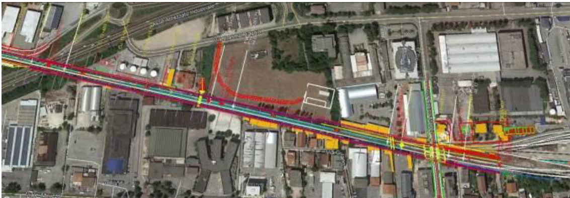
Figura 2-2: Tratti di sede dal km 12+852,056 al km 13+400
