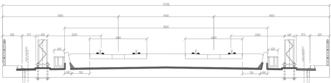
Fig. 56 – Sezione tipo ferroviaria in viadotto a doppio binario
