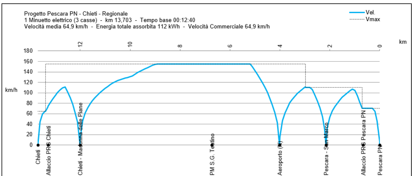
Fig. 29 – Simulazione di marcia. Scenario Raddoppio. Servizio regionale tratta Chieti - Pescara PN. Materiale Ale 501/502 (Minuetto)
