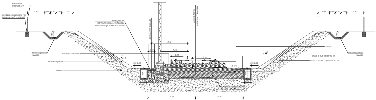
Fig. 54 – Sezione tipo ferroviaria in trincea a singolo binario in rettilfo in corrispondenza del palo TE
