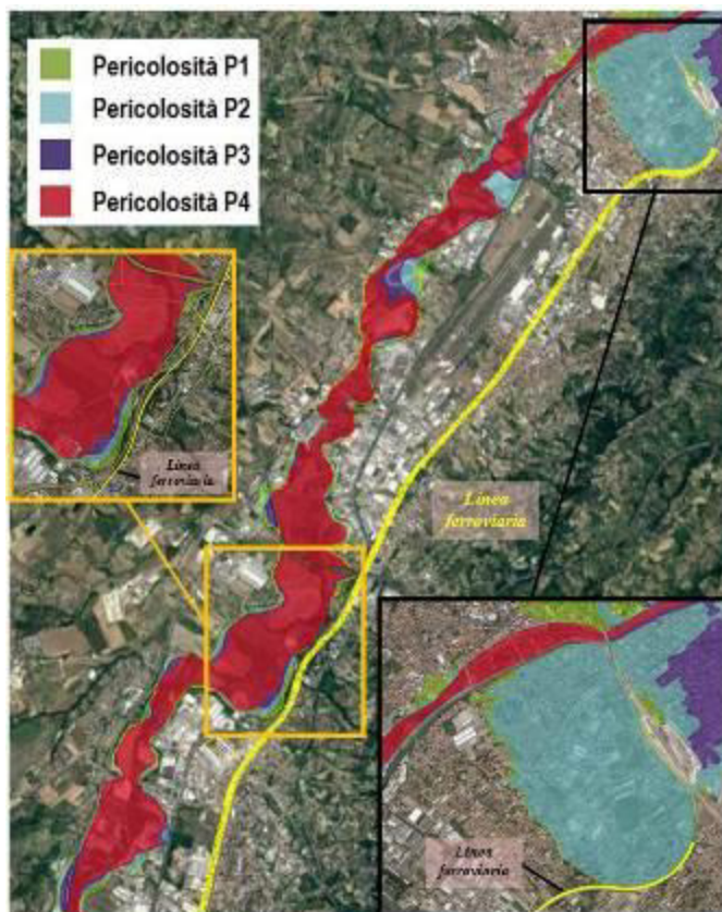
Fig. 38 – Fiume Pescara e linea ferroviaria in progetto: aree a pericolosità idraulica (PSDA).
