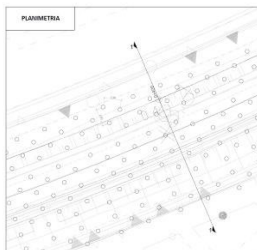
Fig. 35 – Esempio pianta tipo con colonne di deep-mixing
