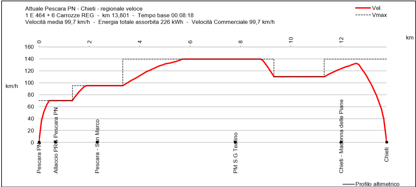
Fig. 26 – Simulazione di marcia. Scenario Attuale. Servizio regionale veloce tratta Pescara PN - Chieti
