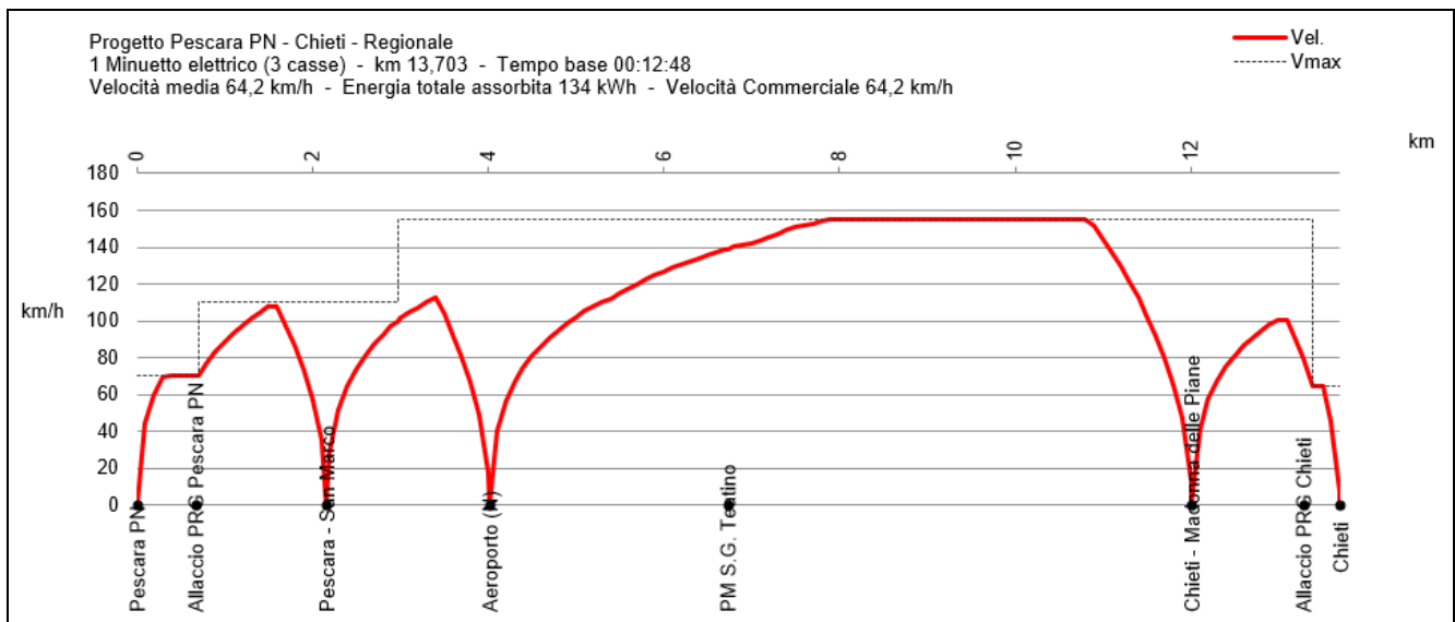
Fig. 28 – Simulazione di marcia. Scenario Raddoppio. Servizio regionale tratta Pescara PN – Chieti. Materiale Ale 501/502 (Minuetto)
