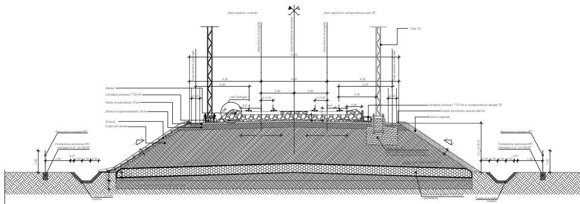
Fig. 44 – Sezione tipo ferroviaria in rilevato a doppio binario (piattaforma in retto) con H_{ri} \leq 6,00 m
