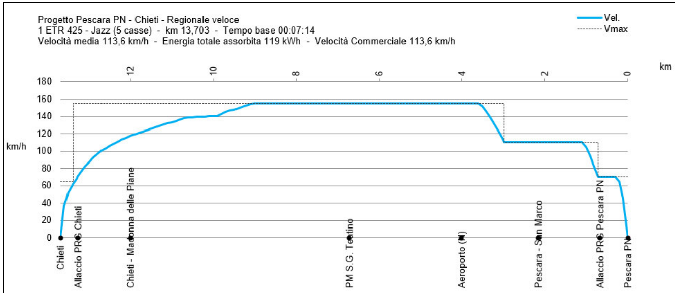
Fig. 33 – Simulazione di marcia. Scenario Raddoppio. Servizio regionale veloce tratta Chieti - Pescara PN. Materiale ETR 425 (Jazz)
