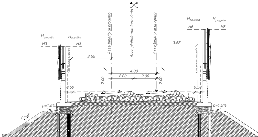
Fig. 61 – Sezione tipo tipologica BA “HS” rettificato con manufatto prefabbricato su rilevato
