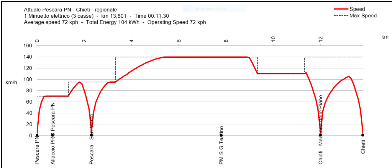
Fig. 24 – Simulazione di marcia. Scenario Attuale. Servizio regionale tratta Pescara PN - Chieti
