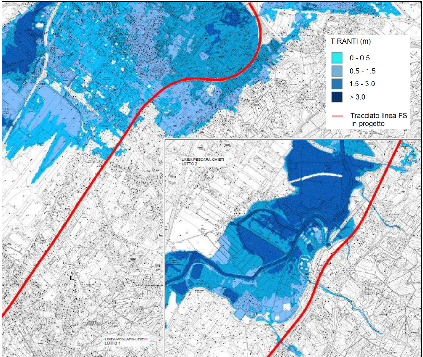
Fig. 41 – Modello idraulico 2D: aree di esondazione (Tr 300 anni) del Fiume Pescara, scenario ante operam.
