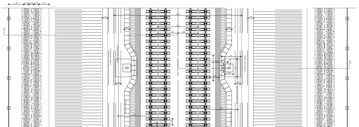
Fig. 50 – Stralcio planimetrico con sezione tipo ferroviaria in trincea a doppio binario in rettilineo
