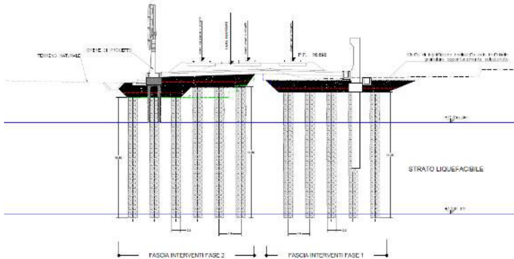
Fig. 36 – Esempio sezione tipo intervento con pali in ghiaia
