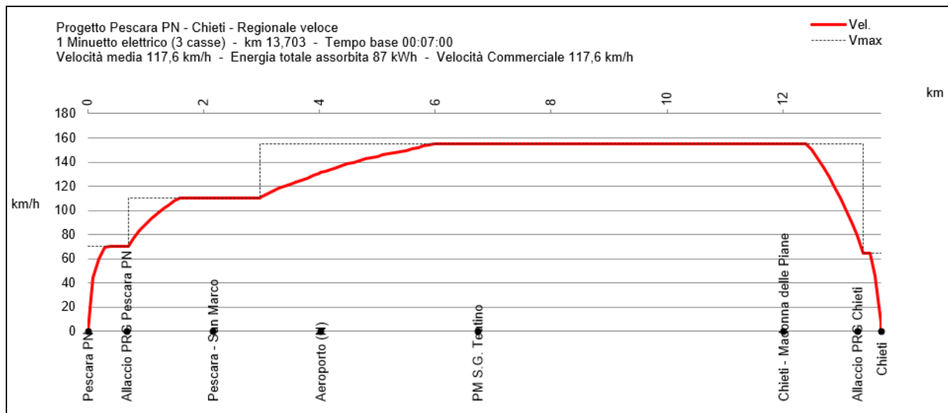
Fig. 30 – Simulazione di marcia. Scenario Raddoppio. Servizio regionale veloce tratta Pescara PN – Chieti. Materiale Ale 501/502 (Minuetto)
