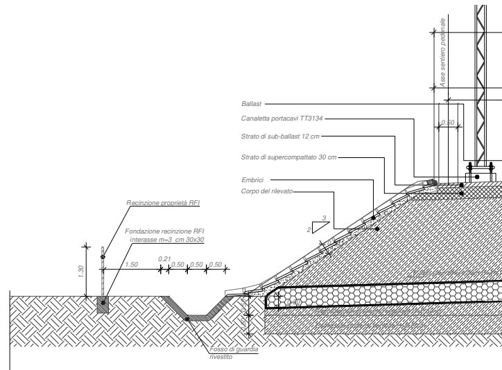
Fig. 46 – Dettaglio alla base del rilevato ferroviario
