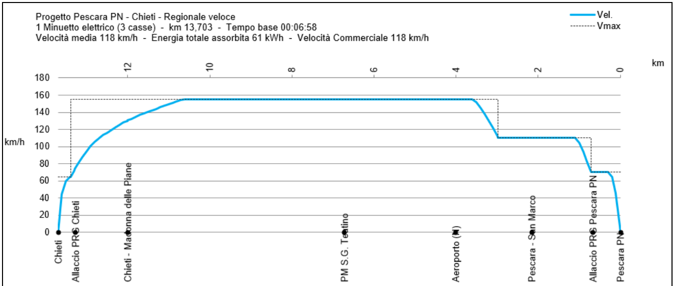
Fig. 31 – Simulazione di marcia. Scenario Raddoppio. Servizio regionale veloce tratta Chieti - Pescara PN. Materiale Ale 501/502 (Minuetto)
