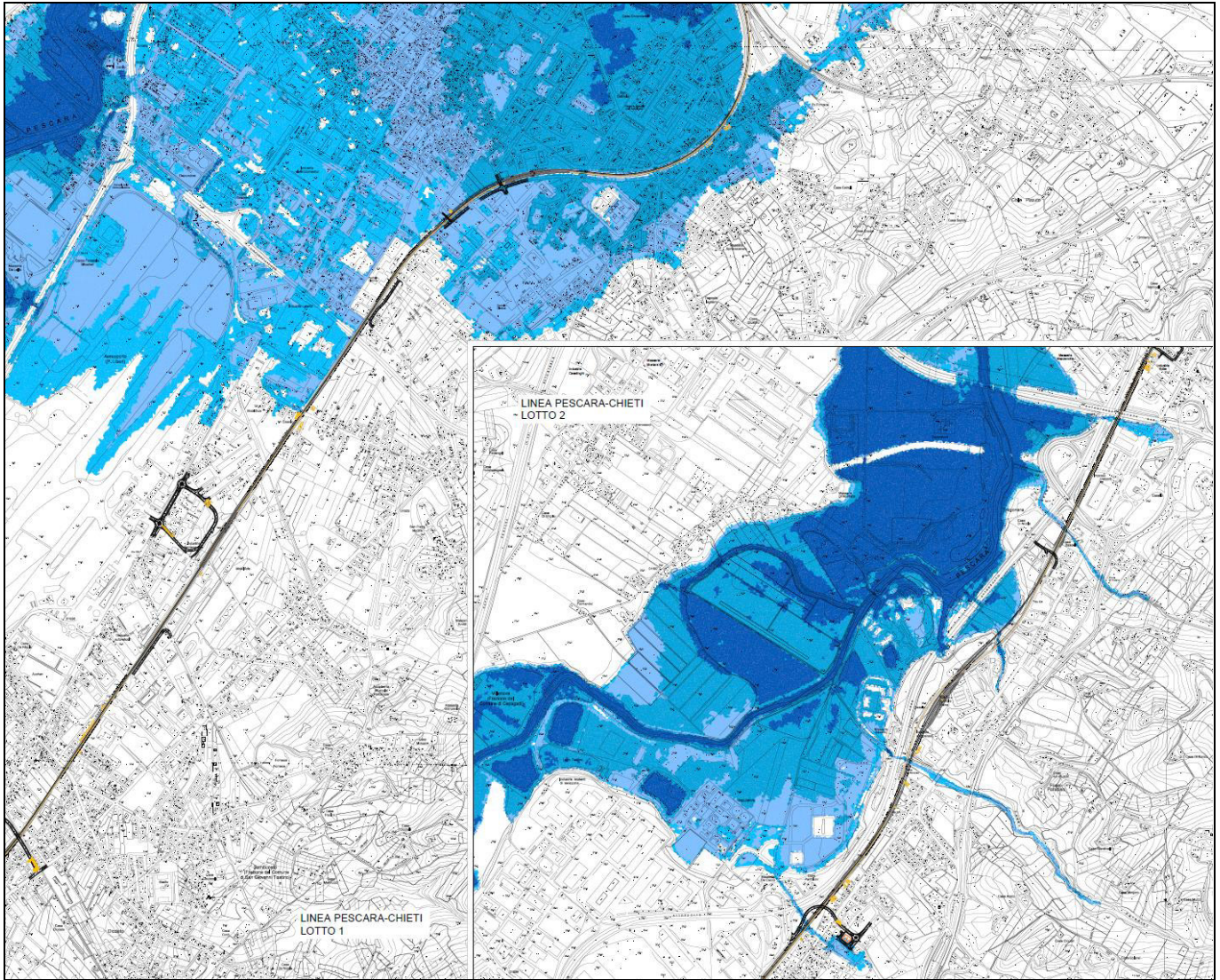
Fig. 42 – Modello idraulico 2D: aree di esondazione (Tr 300 anni) del Fiume Pescara, scenario post operam
