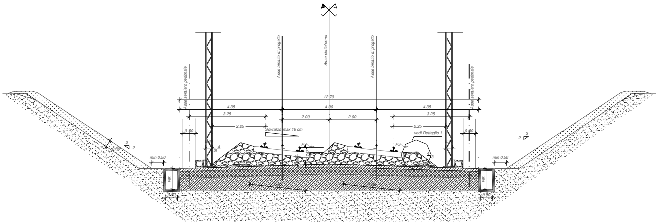
Fig. 51 – Sezione tipo ferroviaria in trincea a doppio binario in curva
