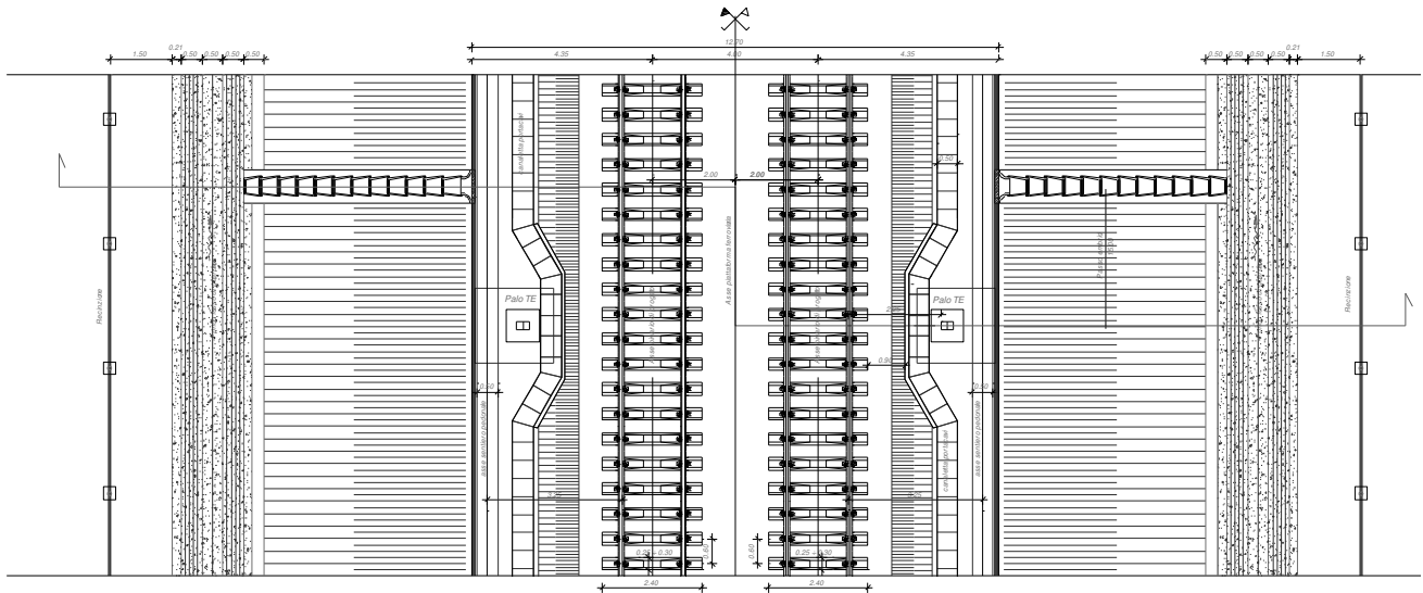
Fig. 45 – Stralcio planimetrico per sezione tipo ferroviaria in rilevato a doppio binario (piattaforma in retto) con H_{ril} \leq 6,00 m
