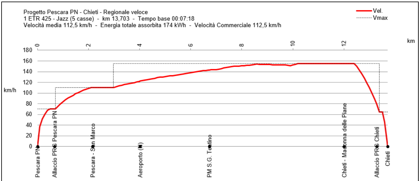
Fig. 32 – Simulazione di marcia. Scenario Raddoppio. Servizio regionale veloce tratta Pescara PN - Chieti. Materiale ETR 425 (Jazz)
