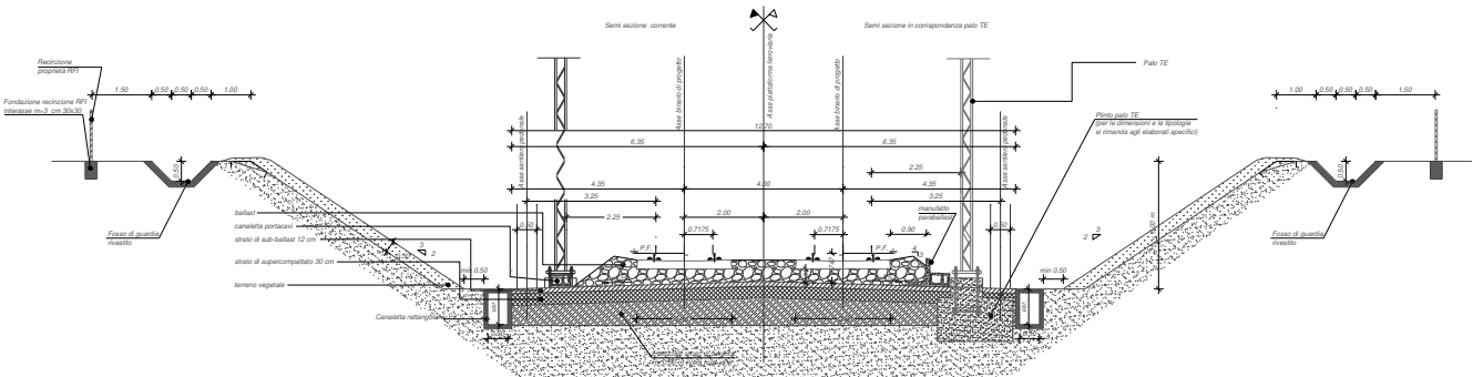
Fig. 49 – Sezione tipo ferroviaria in trincea a doppio binario in rettilineo
