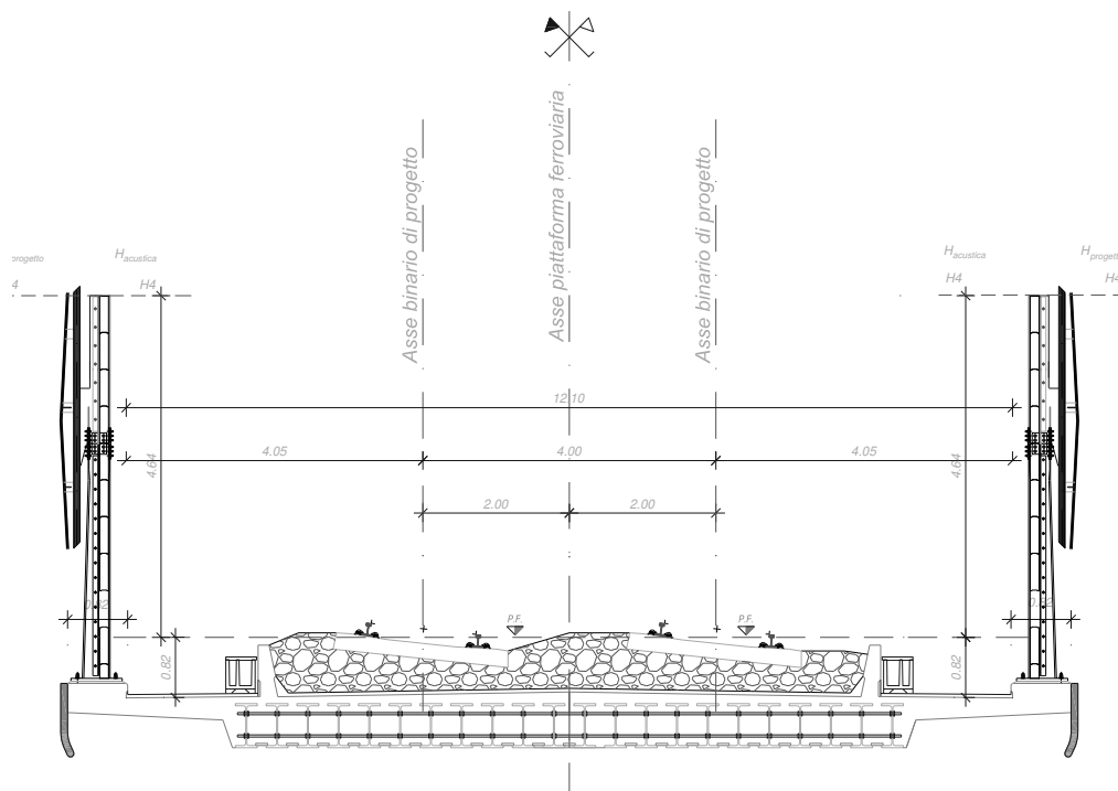
Fig. 63 – Sezione tipo tipologica BA “HS” rettificato su impalcato ferroviario
