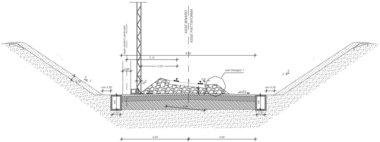
Fig. 55 – Sezione tipo ferroviaria in trincea a singolo binario in curva
