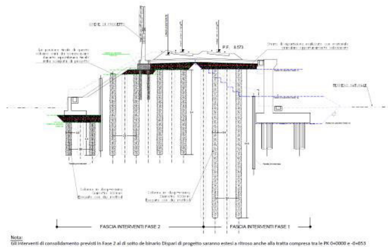
Fig. 34 – Esempio sezione tipo con colonne di deep-mixing
