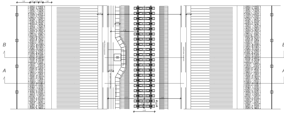
Fig. 53 – Stralcio planimetrico con sezione tipo ferroviaria in trincea a singolo binario in rettilfo
