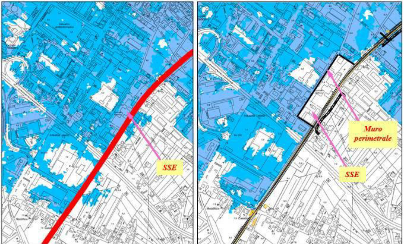
Fig. 43 – Modello idraulico 2D: aree di esondazione (Tr 300 anni) del Fiume Pescara ante operam (a sinistra) e post operam (a destra), in corrispondenza della sottostazione elettrica.
