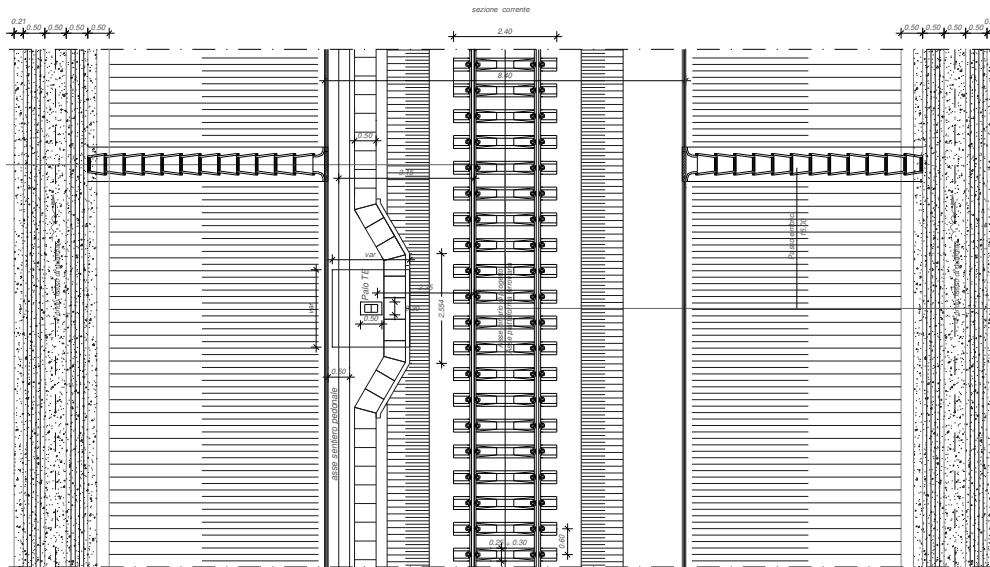
Fig. 48 – Stralcio planimetrico per sezione tipo ferroviaria in rilevato a singolo binario (piattaforma in retto) con H_{ri} \leq 6,00 m
