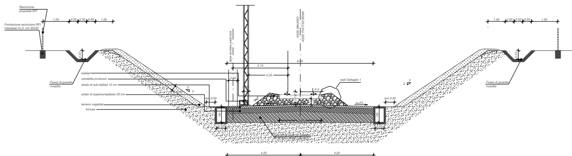
Fig. 52 – Sezione tipo ferroviaria in trincea a singolo binario in rettilineo
