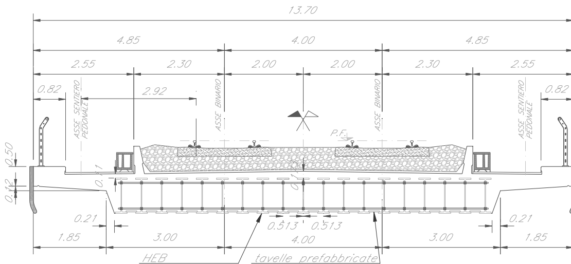
Fig. 58 – Sezione tipo ferroviaria impalcato a travi incorporate a DB
