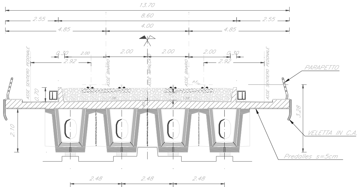
Fig. 59 – Sezione tipo ferroviaria impalcato a 4 cassoncini in CAP a DB
