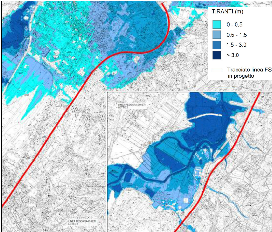
Fig. 39 – Modello idraulico 2D: aree di esondazione (Tr 200 anni) del Fiume Pescara, scenario ante operam.
