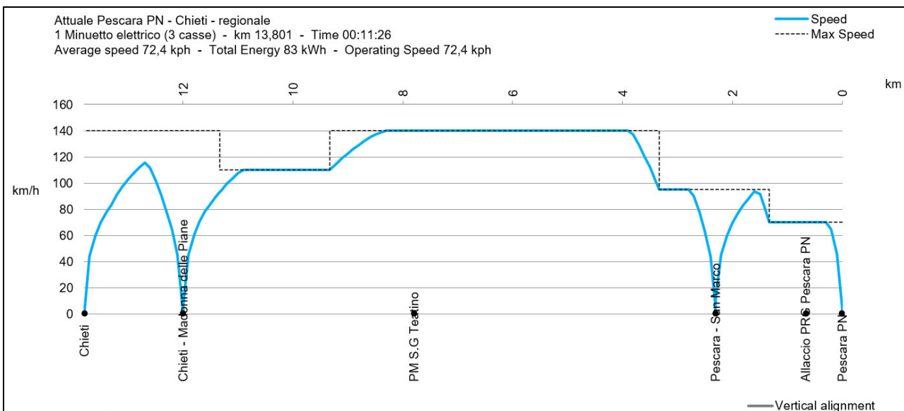
Fig. 25 – Simulazione di marcia. Scenario Attuale. Servizio regionale tratta Chieti - Pescara PN
