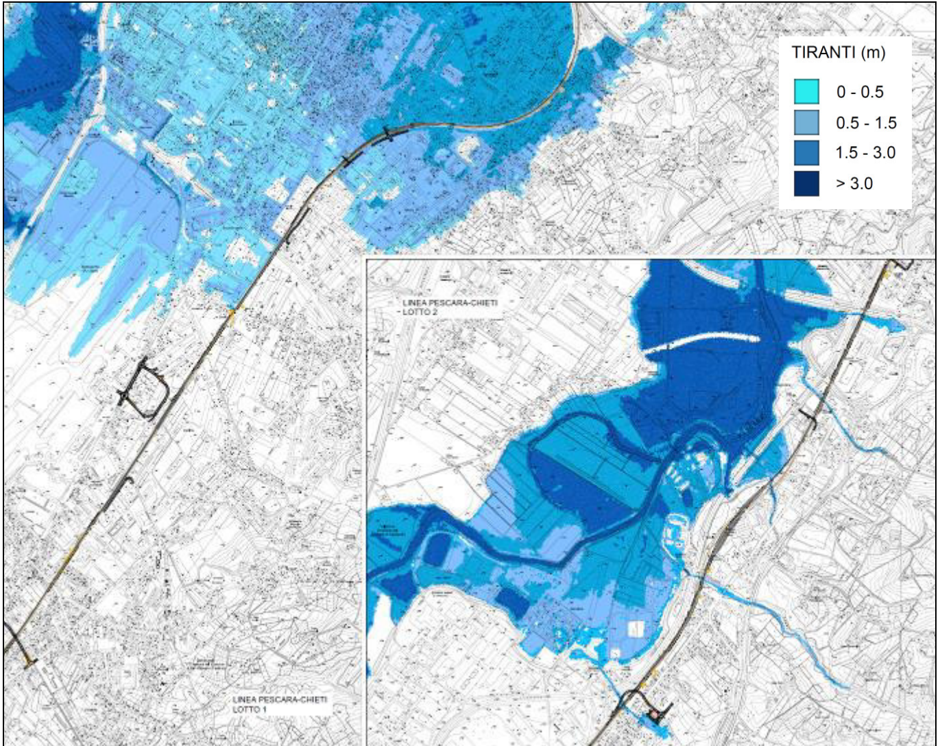
Fig. 40 – Modello idraulico 2D: aree di esondazione (Tr 200 anni) del Fiume Pescara, scenario post operam.
