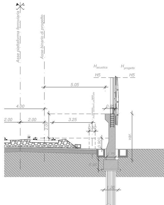
Fig. 62 – Sezione tipo tipologica BA “HS” rettificato senza manufatto prefabbricato fondato su OdS
