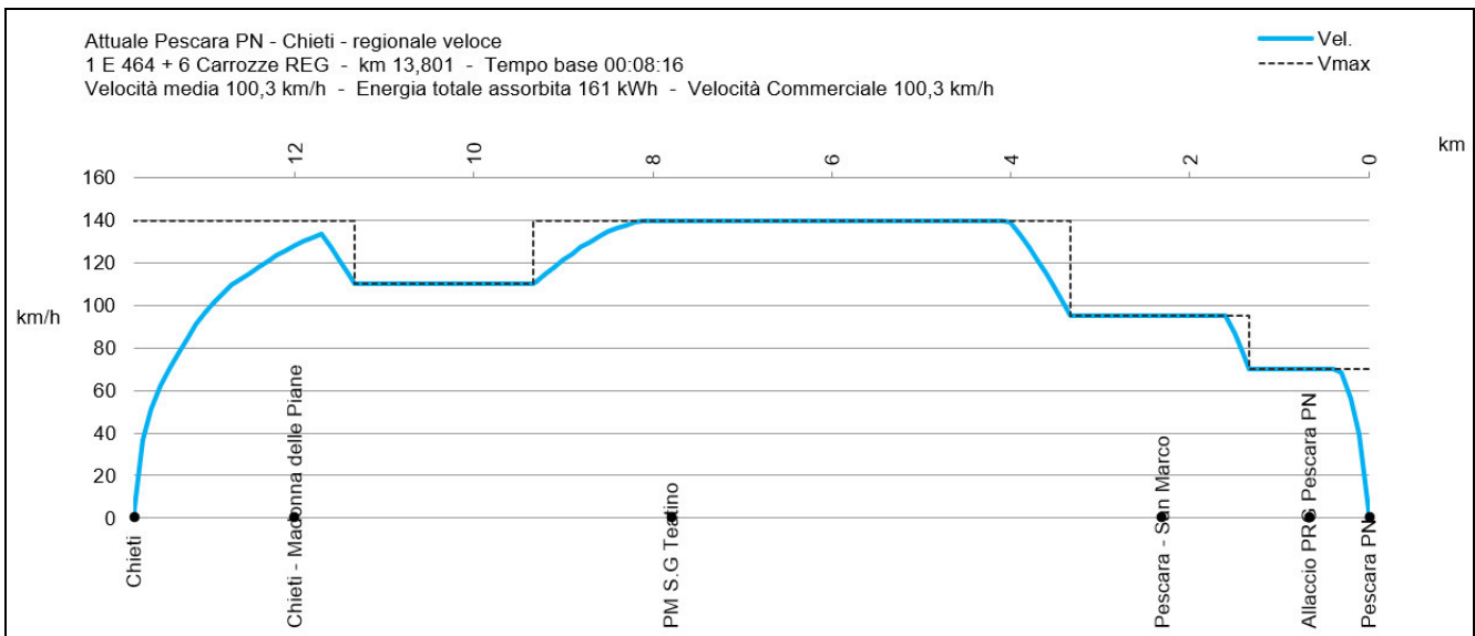
Fig. 27 – Simulazione di marcia. Scenario Attuale. Servizio regionale veloce tratta Chieti - Pescara PN
