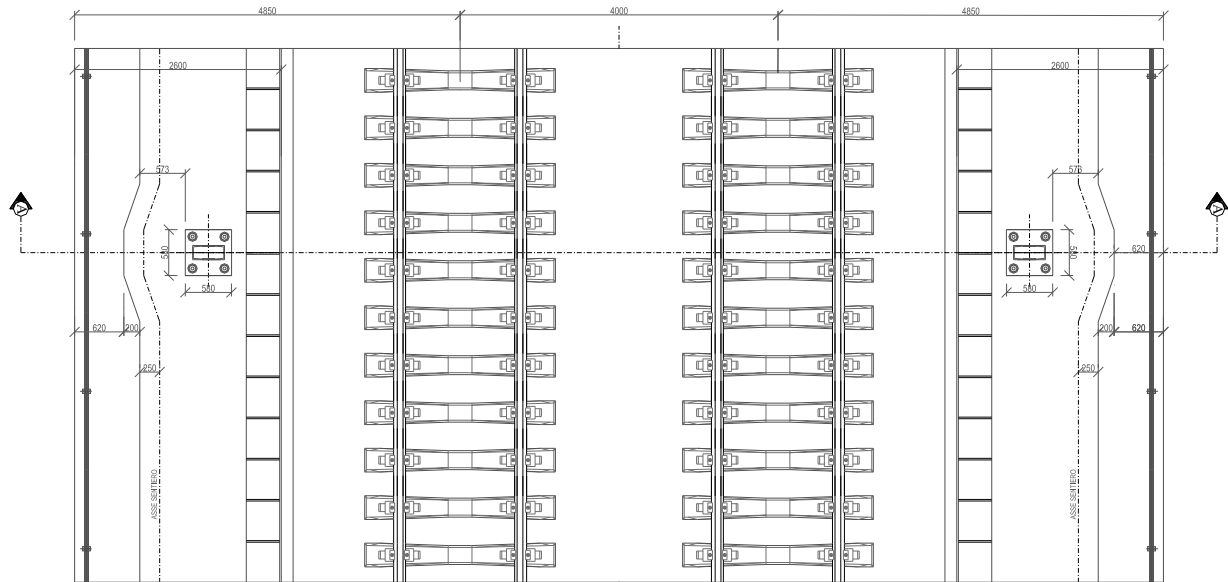
Fig. 57 – Stralcio planimetrico sezione tipo ferroviaria in viadotto a doppio binario
